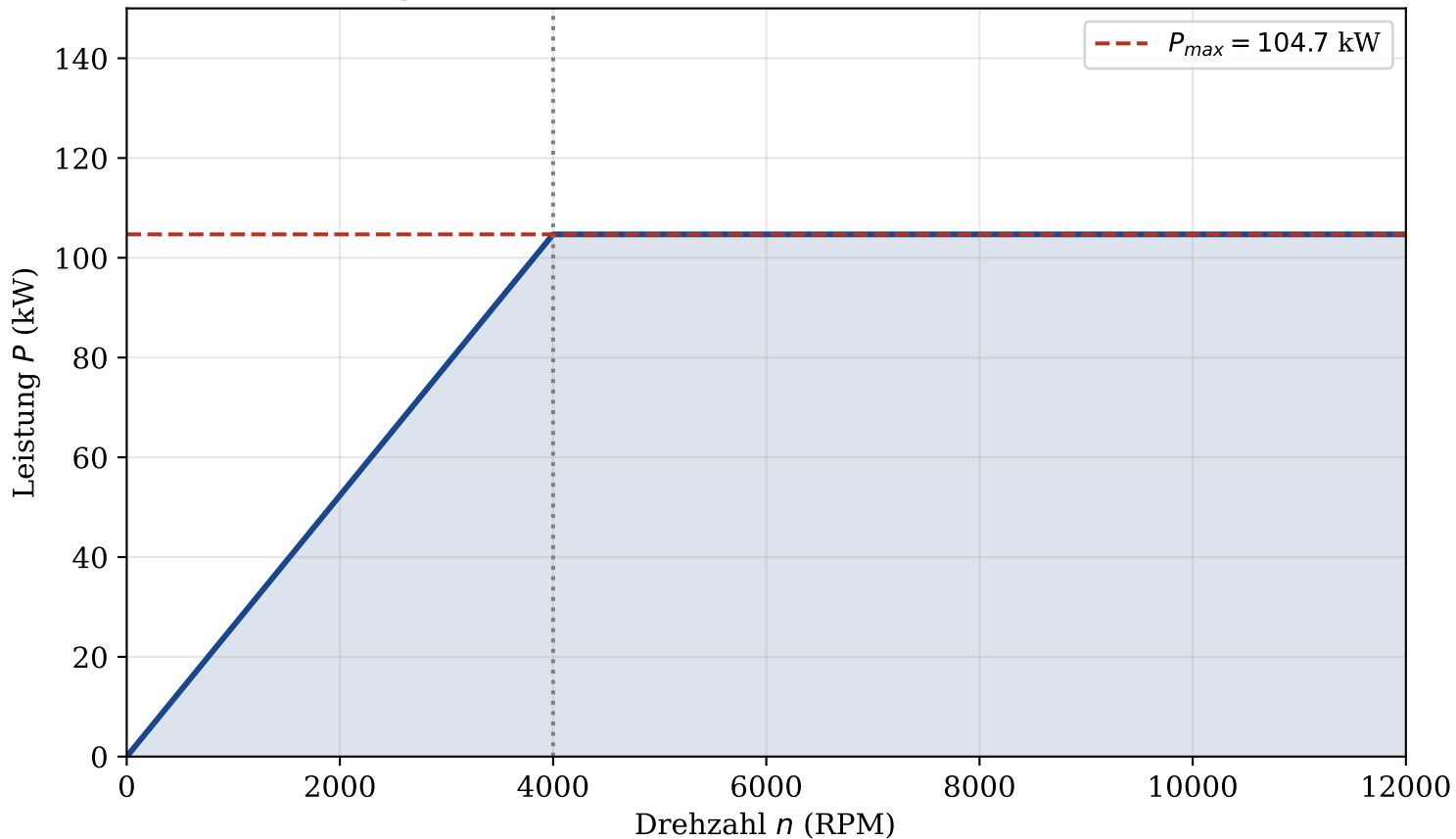
Leistungs-Drehzahl-Kennlinie des PMSM-Traktionsmotors
