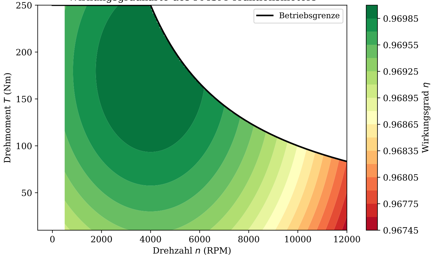
Wirkungsgradkarte des PMSM-Traktionsmotors
