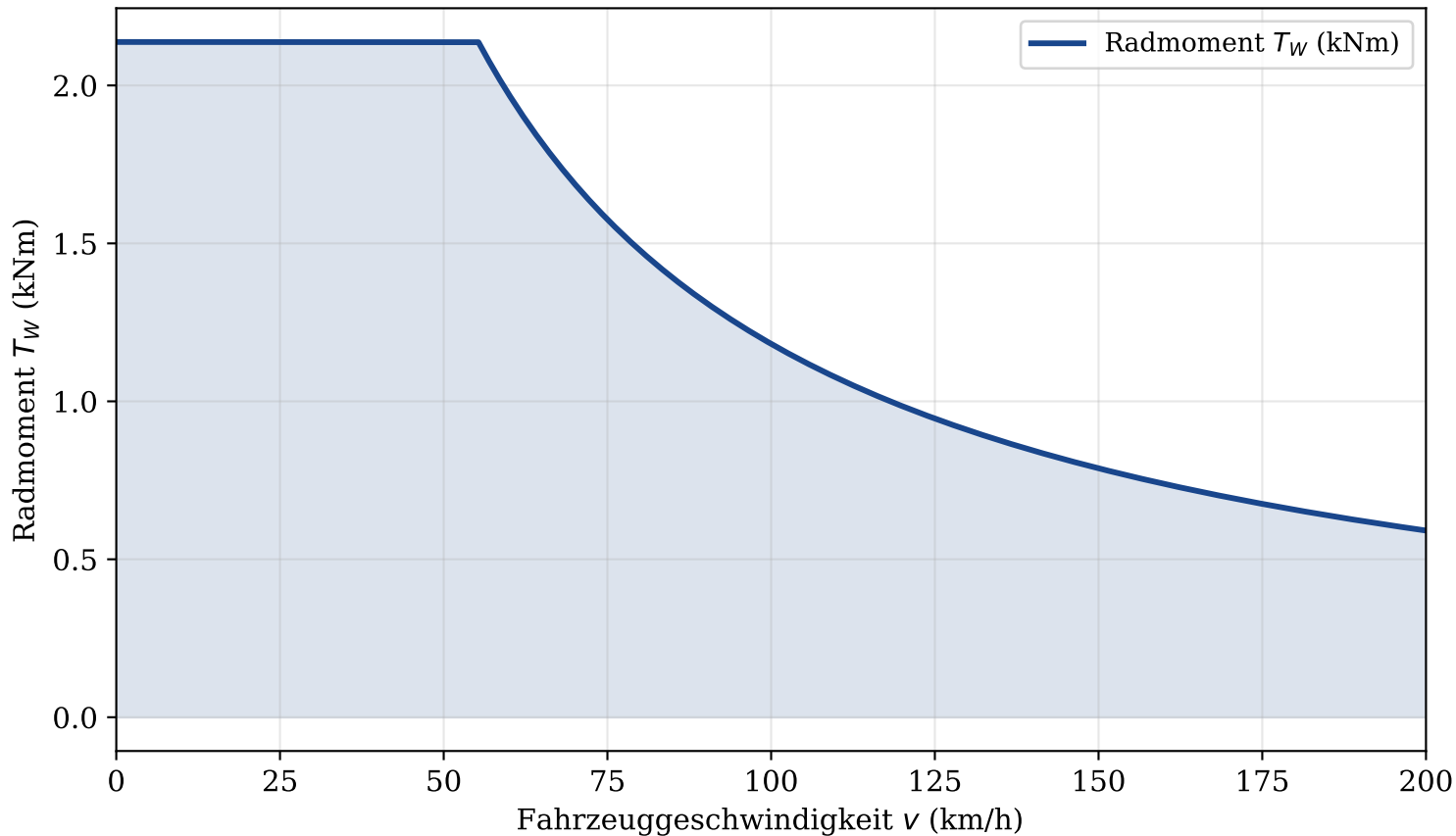
Radmoment über Fahrzeuggeschwindigkeit ( G = 9 , \eta_{DT} = 0.95 )
