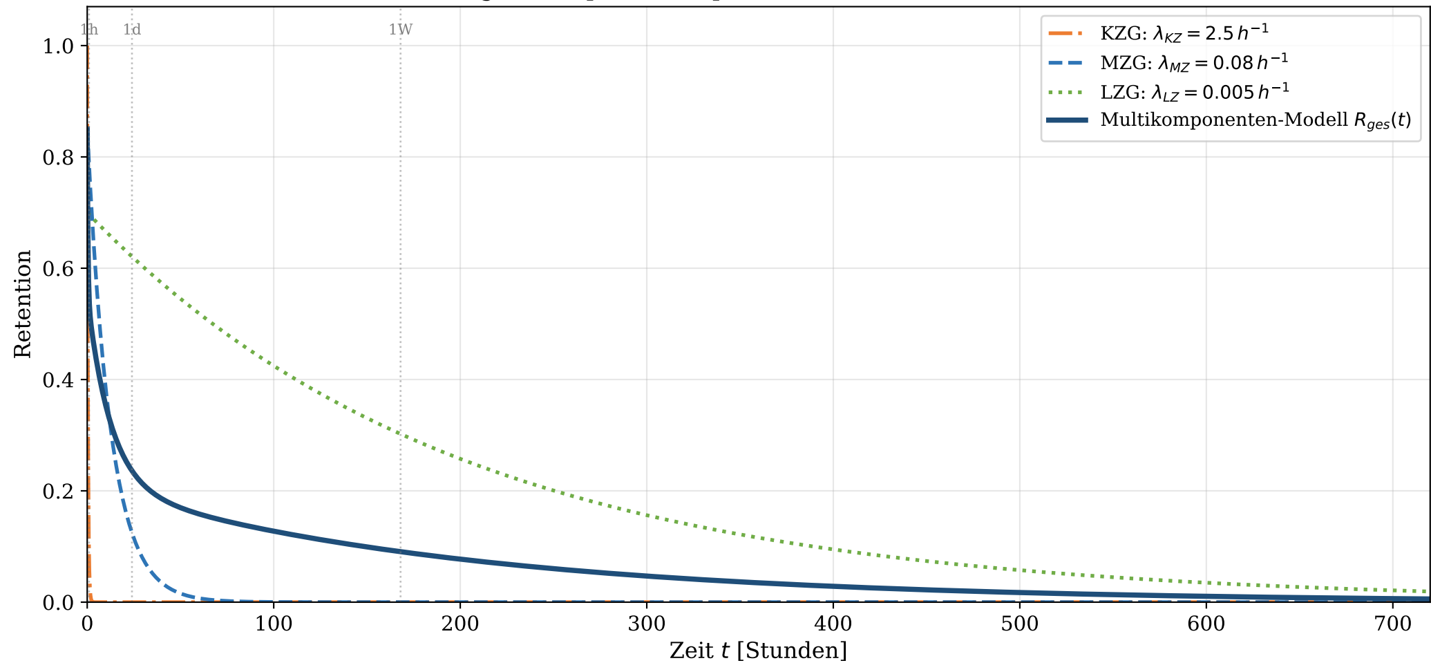
Abbildung 6: Dreiphasen-Exponentialmodell (KZG / MZG / LZG)
