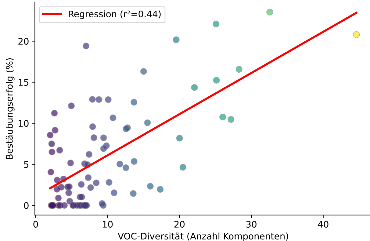
VOC-Diversität vs. Bestäubungsrate
