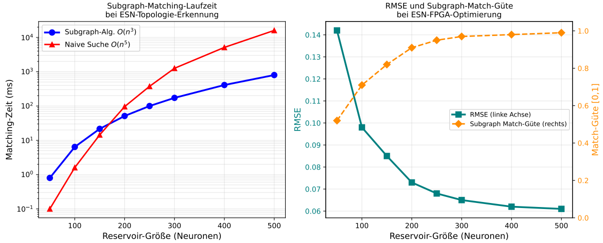
Abbildung 5: Links: Subgraph-Matching-Laufzeit bei ESN-Topologie-Erkennung. Der Subgraph Algorithmus O(n^3) ist gegenüber der naiven Suche O(n^5) bei n = 500 um über zwei Größenordnungen schneller. Rechts: RMSE und Subgraph-Match-Güte in Abhängigkeit von der Reservoir-Größe. Mit wachsender Reservoir-Größe verbessern sich beide Metriken asymptotisch.
