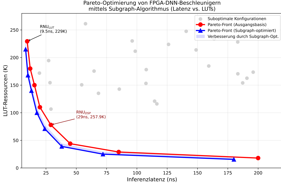
Abbildung 2: Pareto-Front im Latenz-LUT-Raum für FPGA-DNN-Beschleuniger. Die Subgraph-optimierte Partitionierung (blau) verschiebt die Pareto-Front systematisch in Richtung niedrigerer Latenz und geringerem Ressourcenverbrauch. Grau markierte Punkte repräsentieren suboptimale Konfigurationen. Schlüsselkonfigurationen aus [3] sind annotiert.
