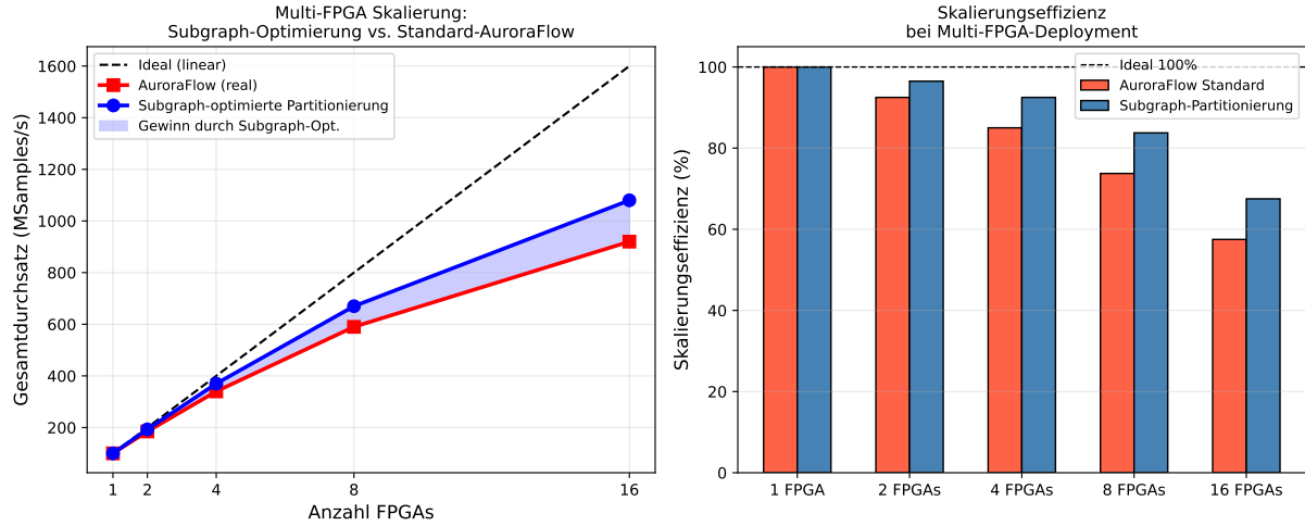
Abbildung 6: Multi-FPGA-Skalierung mit AuroraFlow. Links: Gesamtdurchsatz bei wachsender FPGA-Anzahl. Die Subgraph-optimierte Partitionierung (blau) übertrifft den Standard-AuroraFlow (rot) konsistent. Rechts: Skalierungseffizienz in Prozent der idealen linearen Skalierung. Bei 16 FPGAs erreicht die Subgraph-Methode 67,5 % Effizienz gegenüber 57,5 %.
