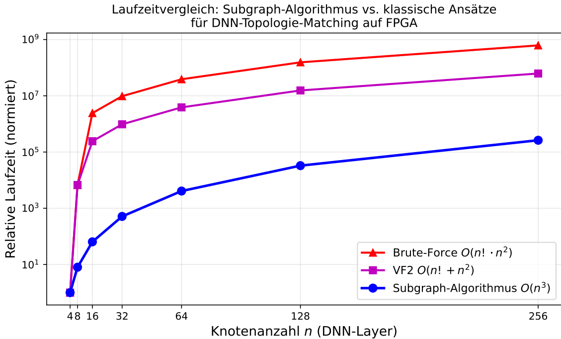
Abbildung 1: Laufzeitvergleich des Subgraph Algorithmus O(n^3) gegenüber Brute-Force O(n! \cdot n^2) und VF2 O(n! + n^2) für DNN-Topologie-Matching auf FPGA-Hardware. Die logarithmische Skalierung verdeutlicht den exponentiellen Vorteil für n \geq 16 .
