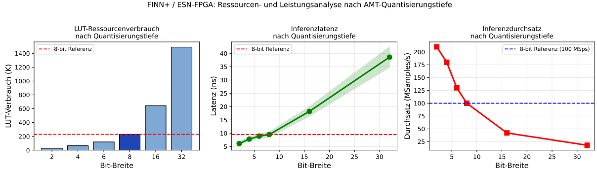
Abbildung 3: Ressourcen- und Leistungsanalyse nach Quantisierungstiefe für FINN+/ESN-FPGA. Links: LUT-Verbrauch wächst superlinear mit der Bit-Breite. Mitte: Latenz nimmt mit steigender Bit-Breite zu. Rechts: Durchsatz sinkt erwartungsgemäß. Die 8-bit Konfiguration (roter Strich) stellt den Referenzpunkt aus [3] dar.
