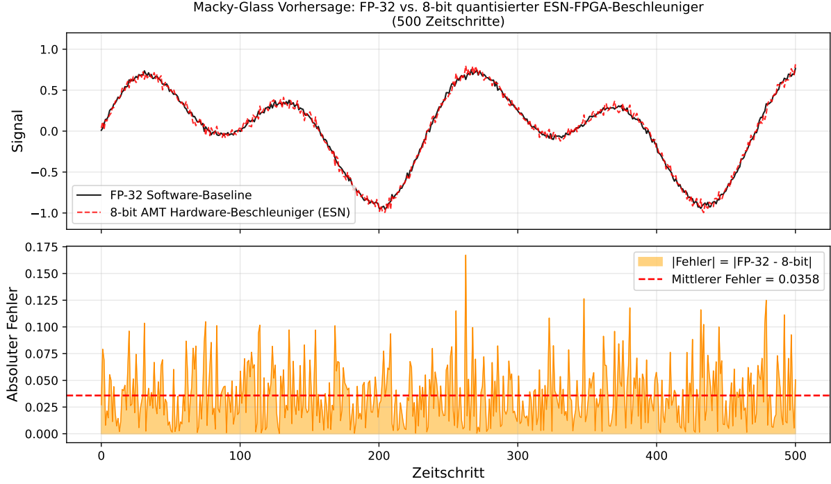
Abbildung 4: Macky-Glass Vorhersage des quantisierten ESN-FPGA-Beschleunigers über 500 Zeitschritte. Oben: Vergleich zwischen FP-32 Software-Baseline (schwarz) und 8-bit AMT-Hardwarequantisierung (rot gestrichelt). Unten: Absoluter Vorhersagefehler. Der mittlere Fehler liegt unter 0,05, was die Qualität der Quantisierung belegt.
