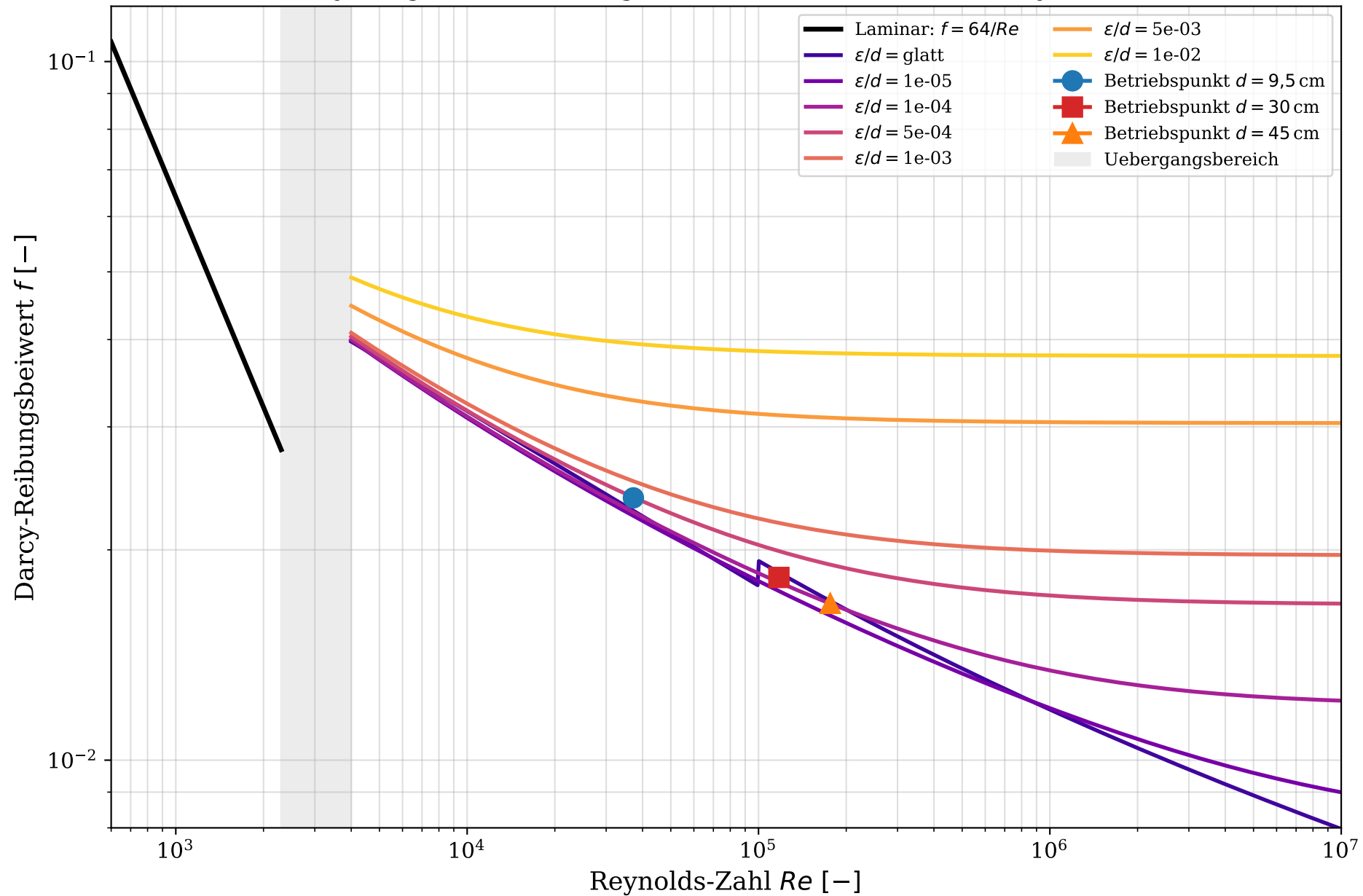
Moody-Diagramm: Reibungsbeiwert als Funktion der Reynolds-Zahl
