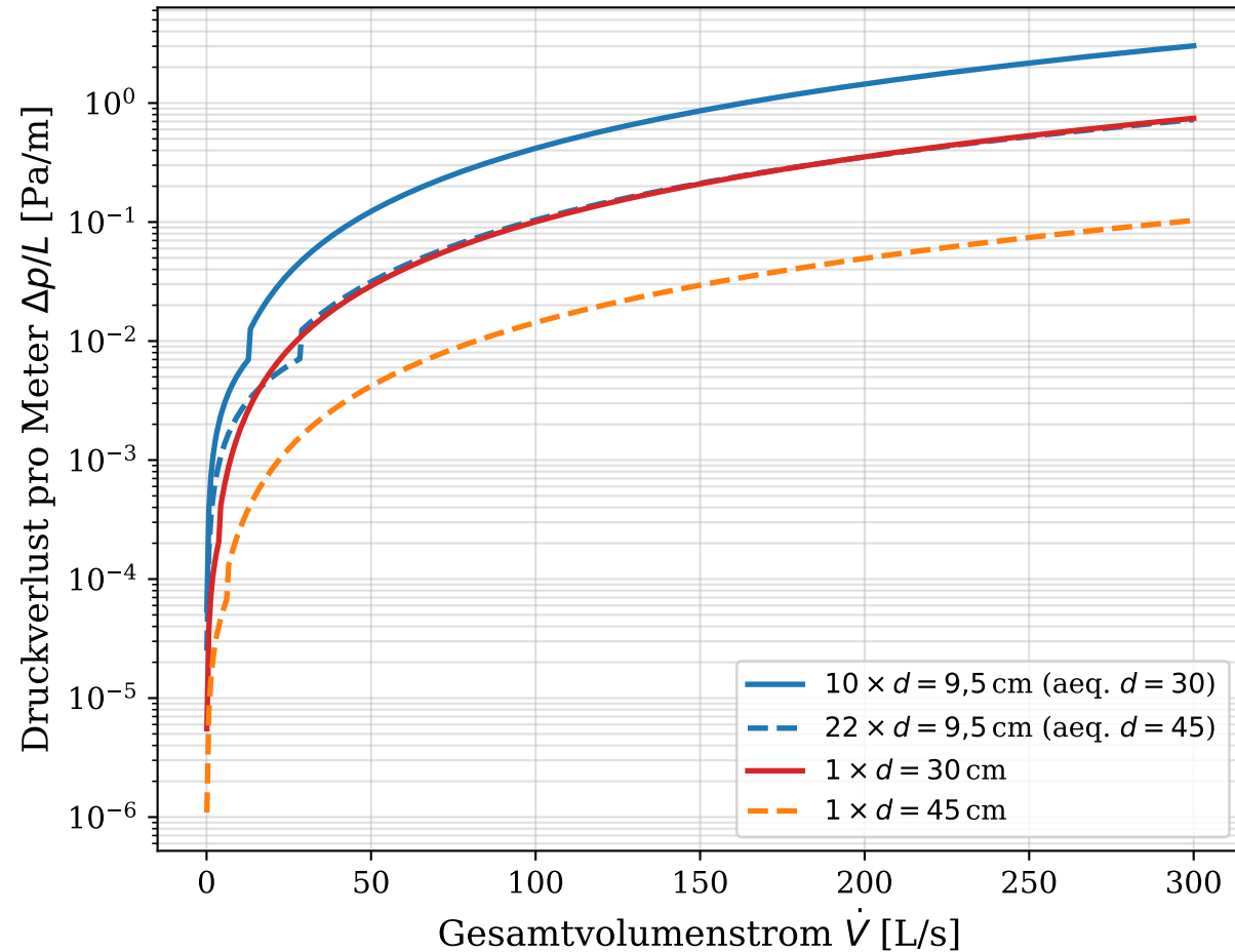
Parallelnetz vs. Einzelrohr (gleiche Gesamtquerschnittsfläche)
