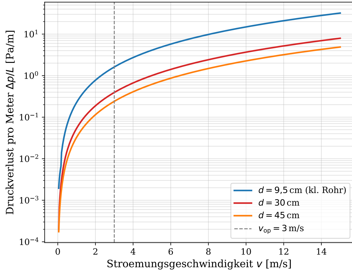
Einzelrohr-Druckverlust
