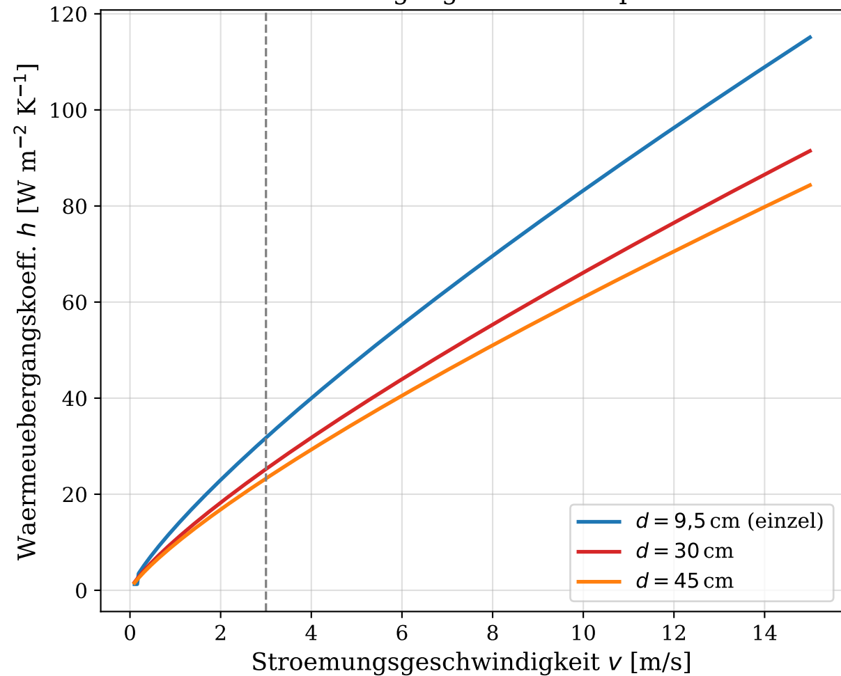
Waermeuebergangskoeffizient pro Rohr
