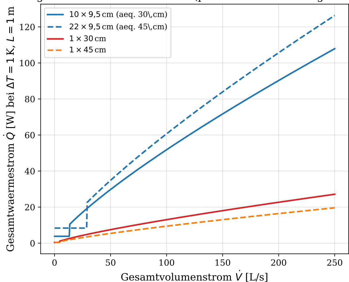
Vergleich Gesamtwarmestrom (parallele kl. vs. eines gr. Rohrs)
