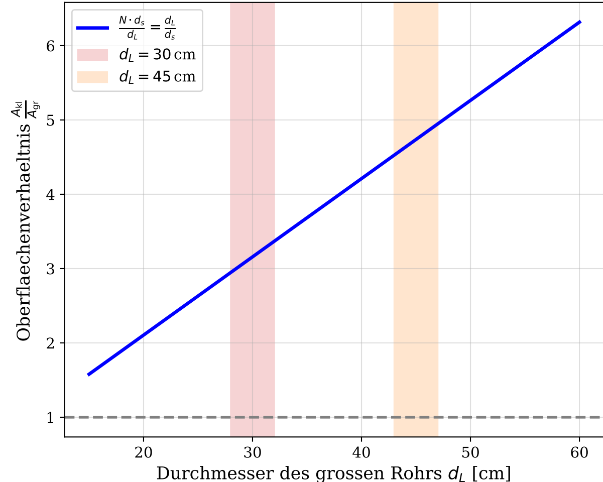
Oberflaechenverhaeltnis der Parallelrohre vs. Einzelrohr
