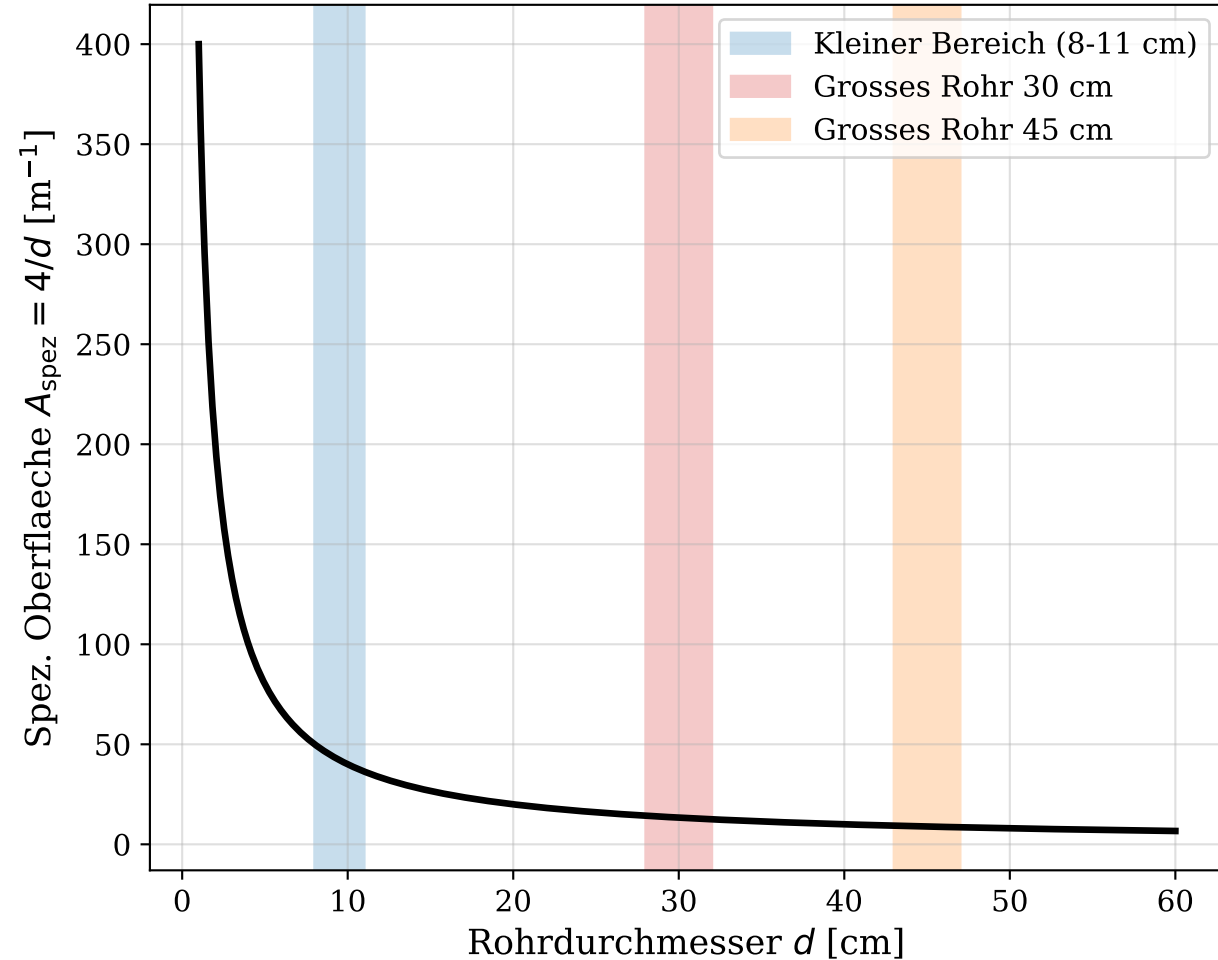
Spezifische Wandoberflaeche pro Gasvolumen
