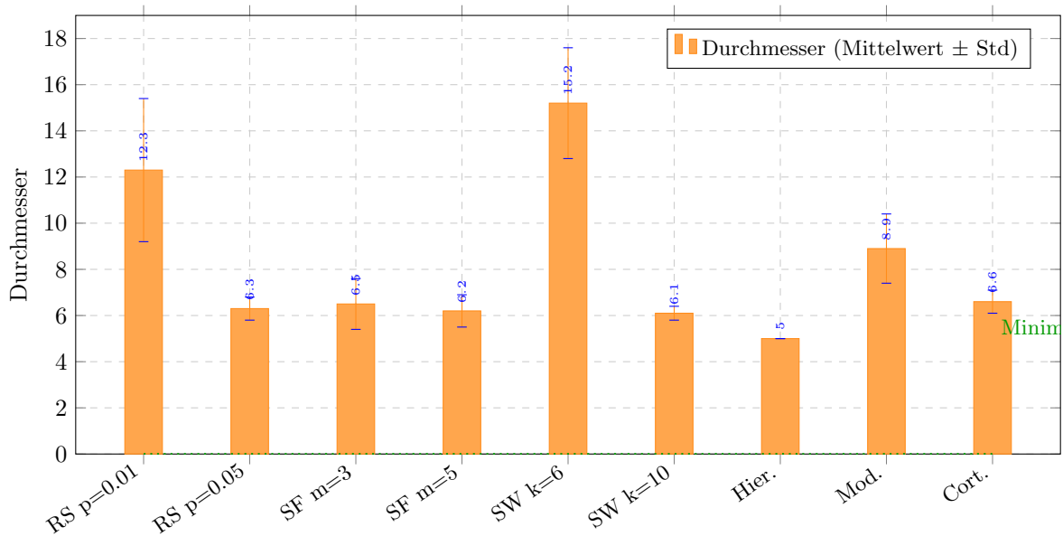
Durchmesser-Verteilung über Graphtypen
