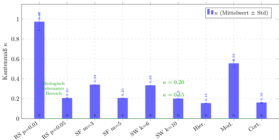
Kantenmaß-Verteilung über Graphtypen
