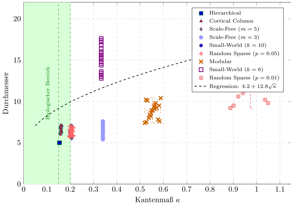
Scatter-Plot: Kantenmaß \kappa versus Durchmesser
