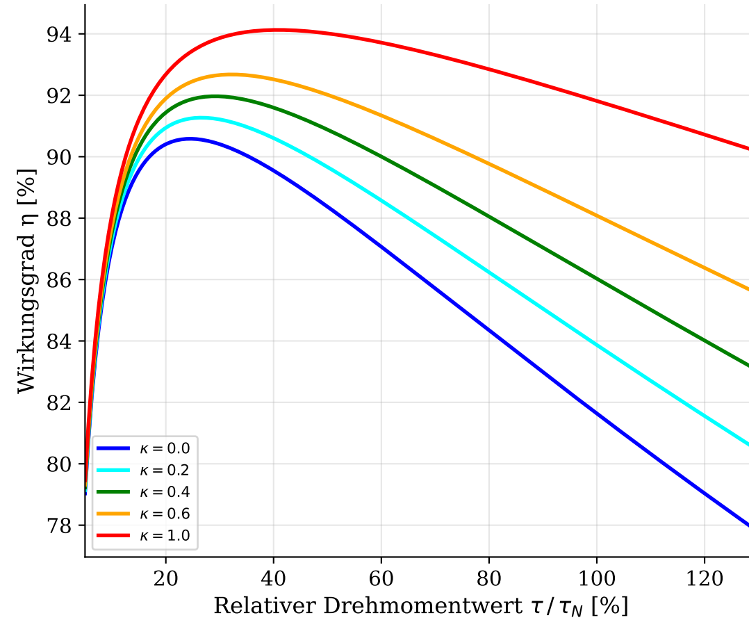
\eta -Kennlinie für verschiedene gravitative Entlastungsgrade \kappa
