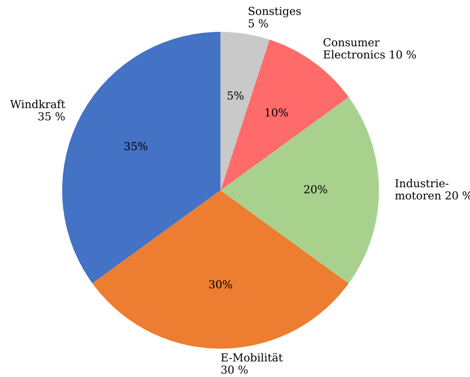
NdFeB-Verbrauch nach Sektor (global, ca. 2024)
