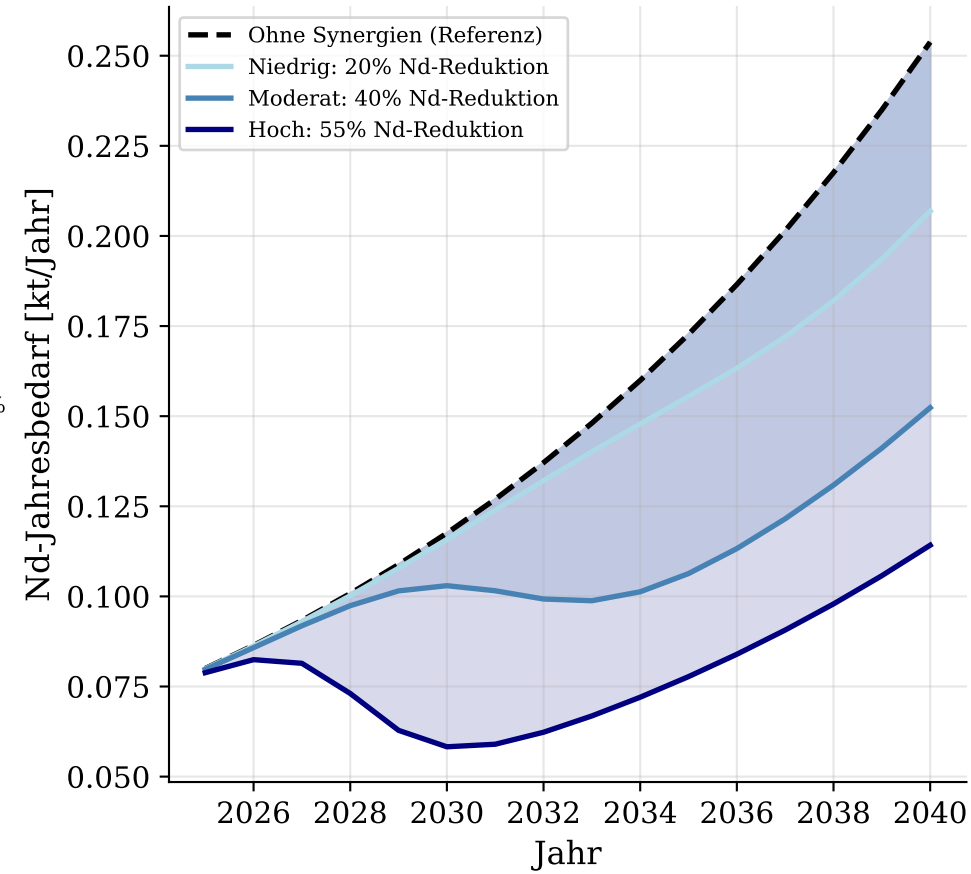
Prognostizierter Nd-Jahresbedarf mit/ohne Synergiekonzepte
