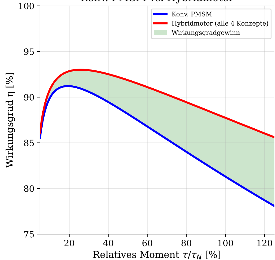
Vollst. Wirkungsgradkennlinie: Konv. PMSM vs. Hybridmotor
