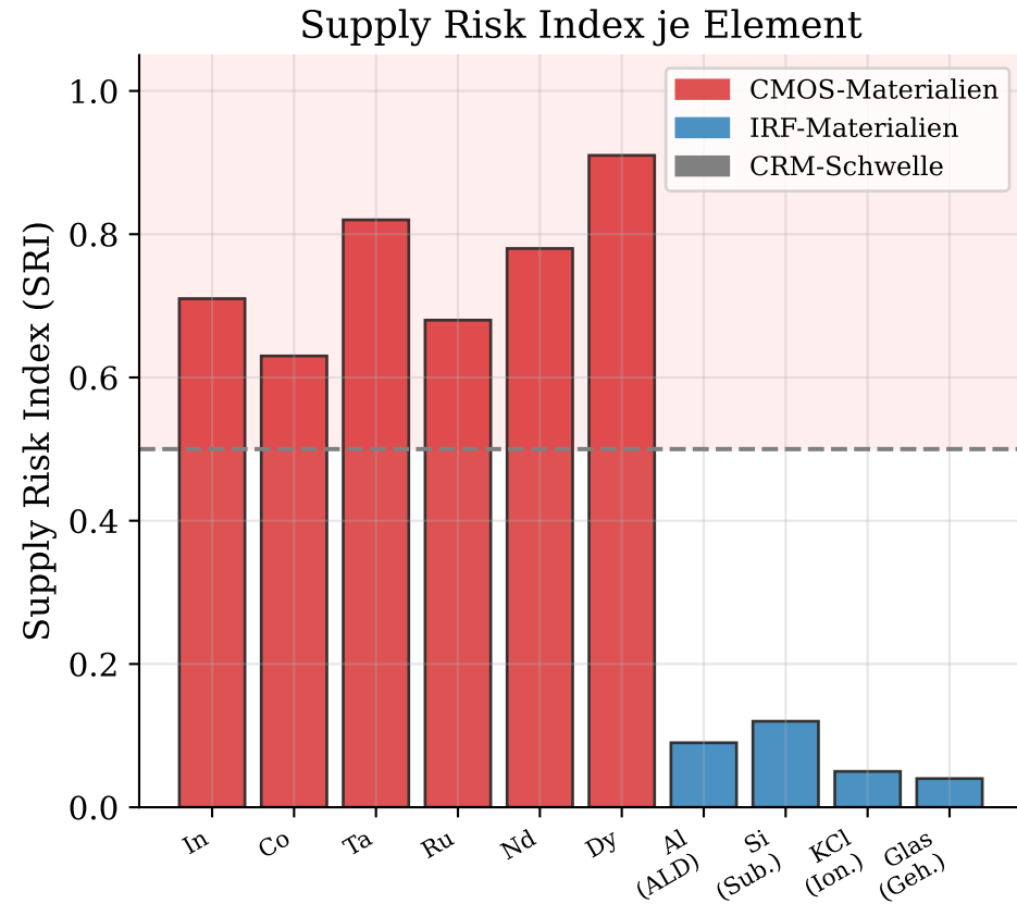
Abbildung 17 - Kritische Materialien: CMOS- vs. IRF-Architektur
