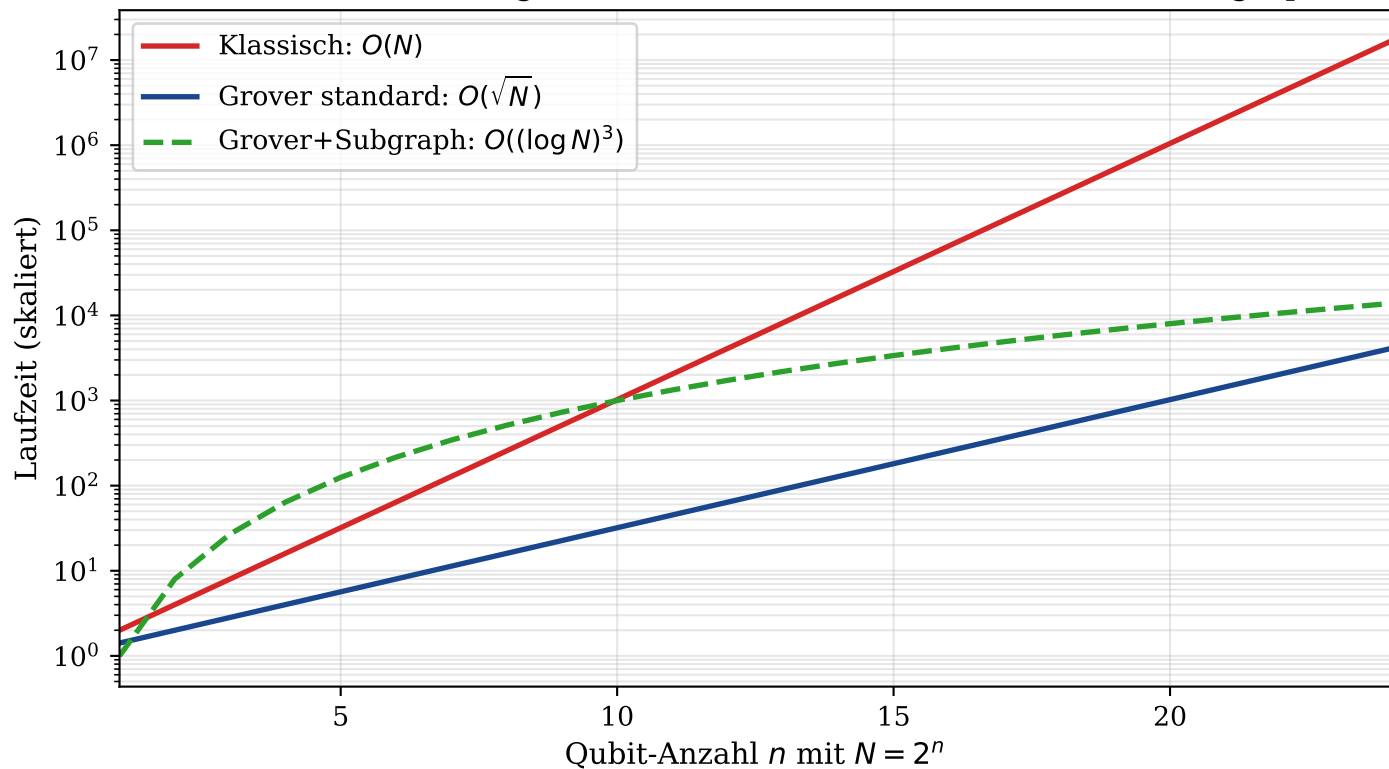
Plot 1 — Laufzeitvergleich: Klassisch vs. Grover vs. Grover+Subgraph
