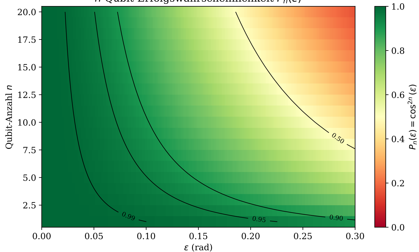
n -Qubit-Erfolgswahrscheinlichkeit P_n(\varepsilon)
