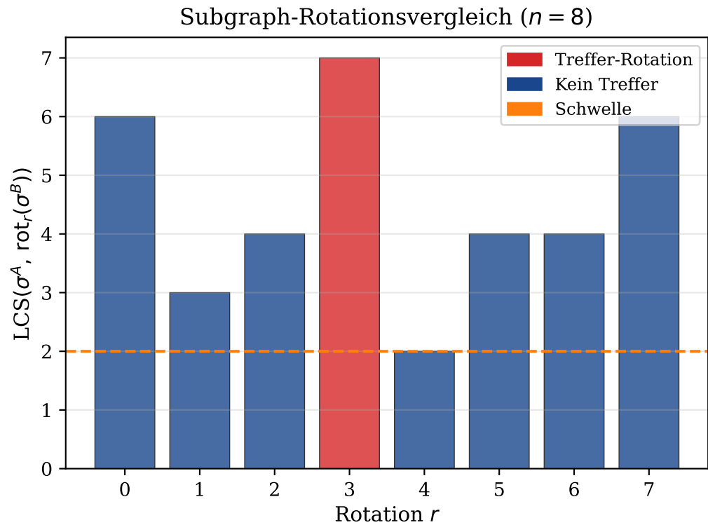
Plot 6 — Grover-Iteration als zyklische Subgraph-Rotation
