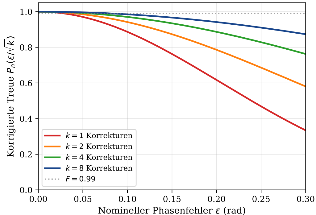
Subgraph-Fehlerkorrektur ( n = 12 Qubits)
