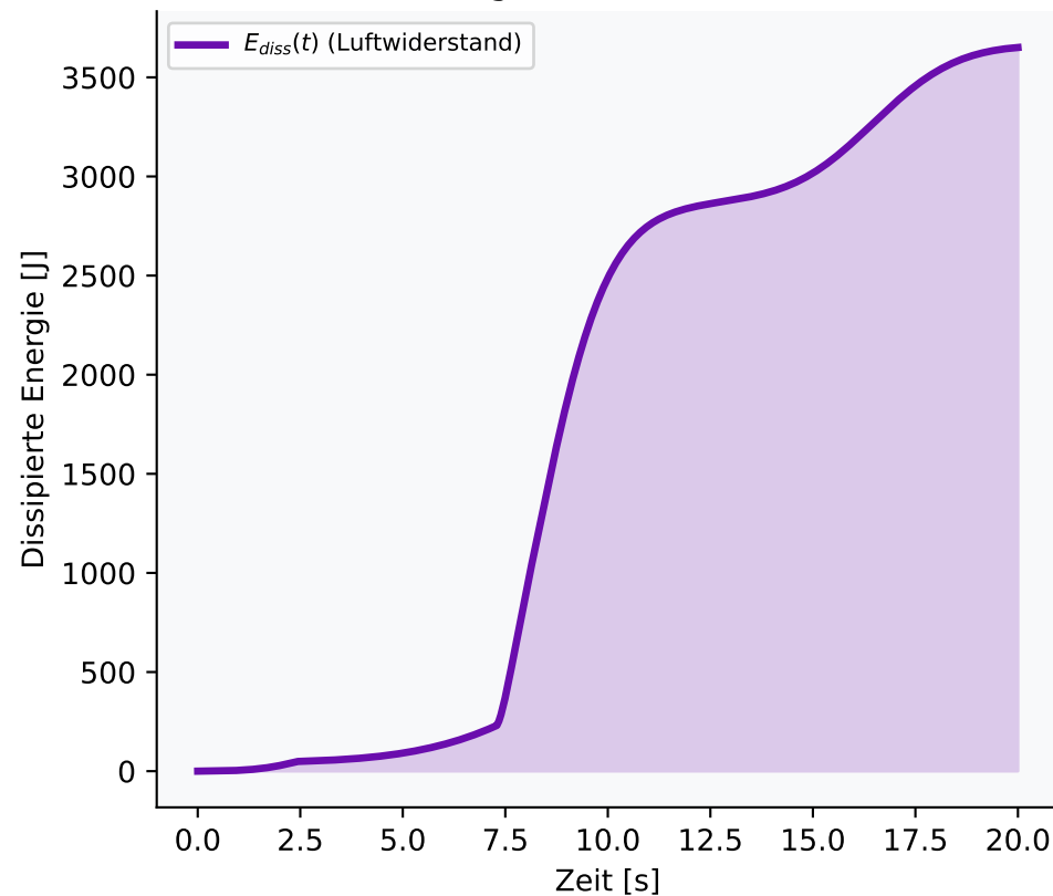
Verlustenergie durch Luftwiderstand
