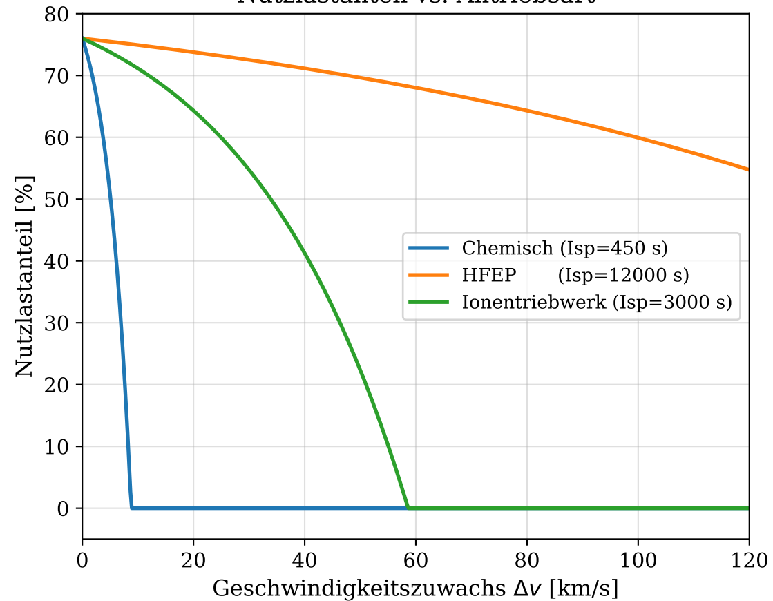
Nutzlastanteil vs. Antriebsart
