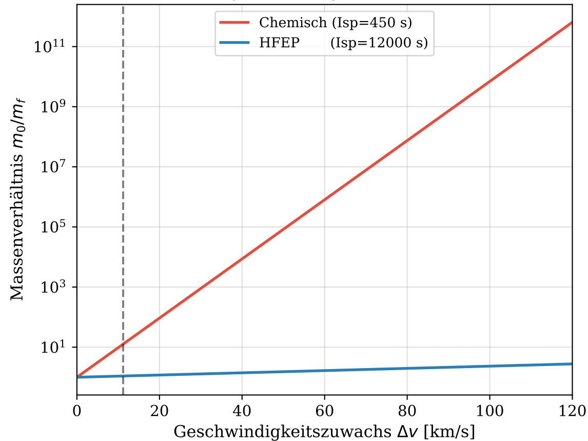
Tsiolkovsky-Gleichung: Massenverhältnis
