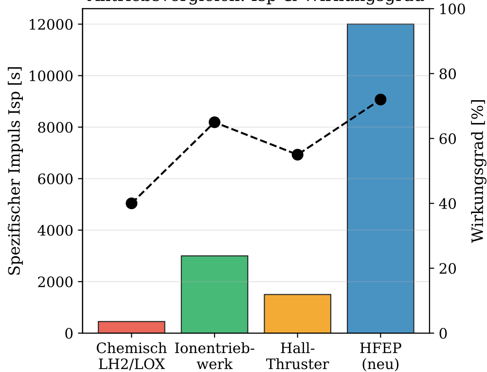
Antriebsvergleich: Isp &amp; Wirkungsgrad
