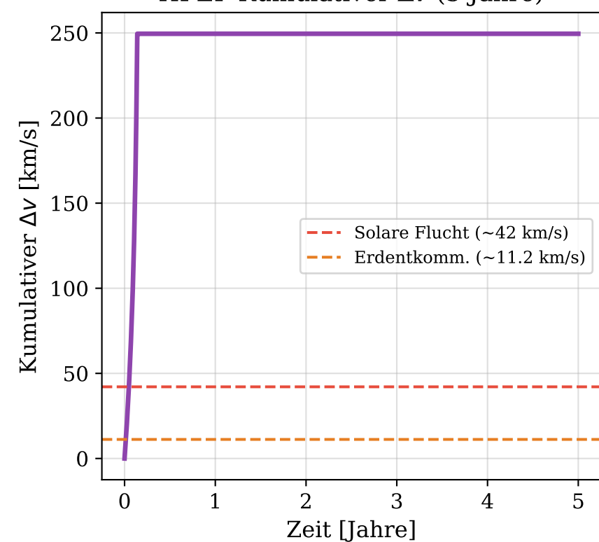
HFEP Kumulativer \Delta v (5 Jahre)
