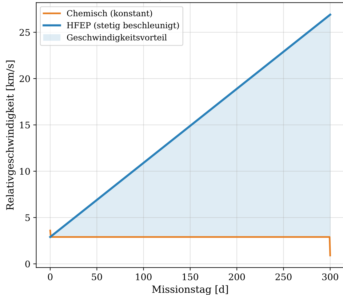
Geschwindigkeitsprofil der Mission
