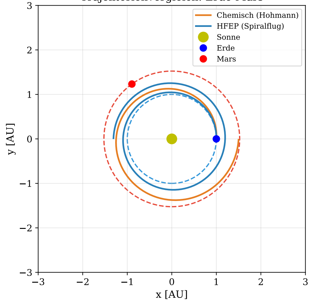
Trajektorienvergleich: Erde-Mars
