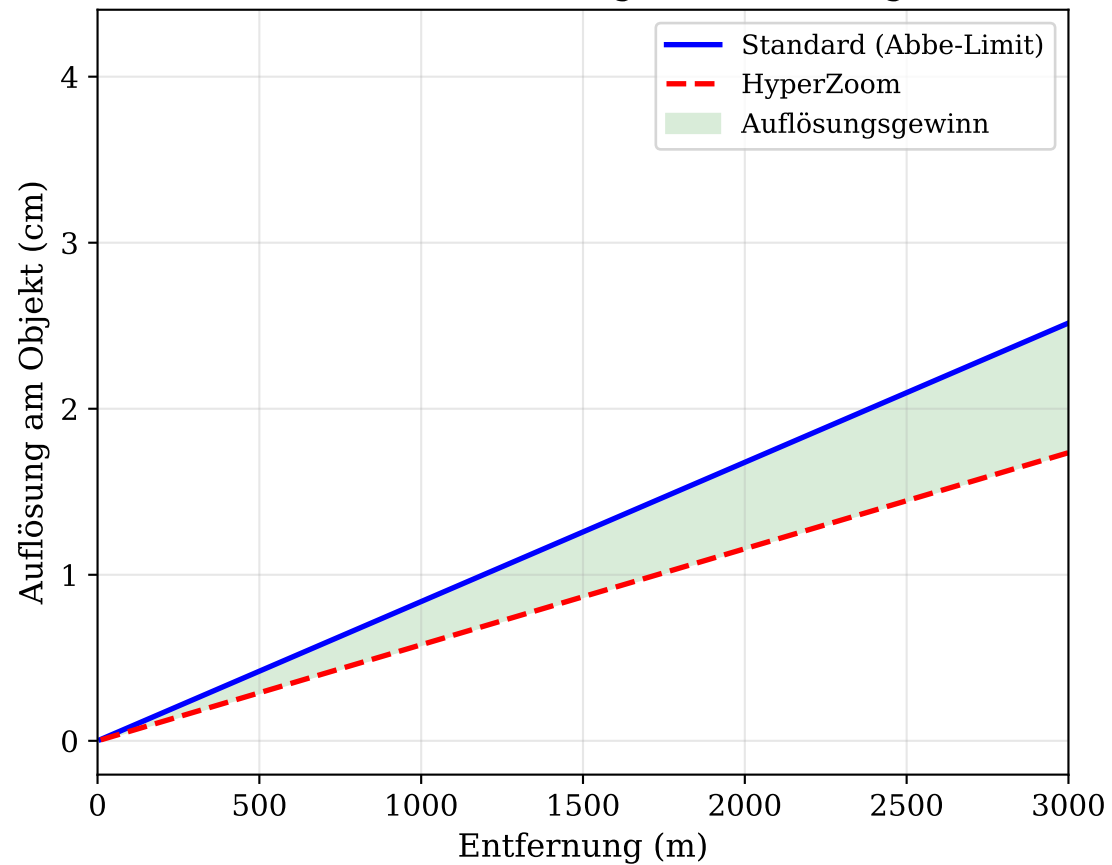
Räumliche Auflösung vs. Entfernung
