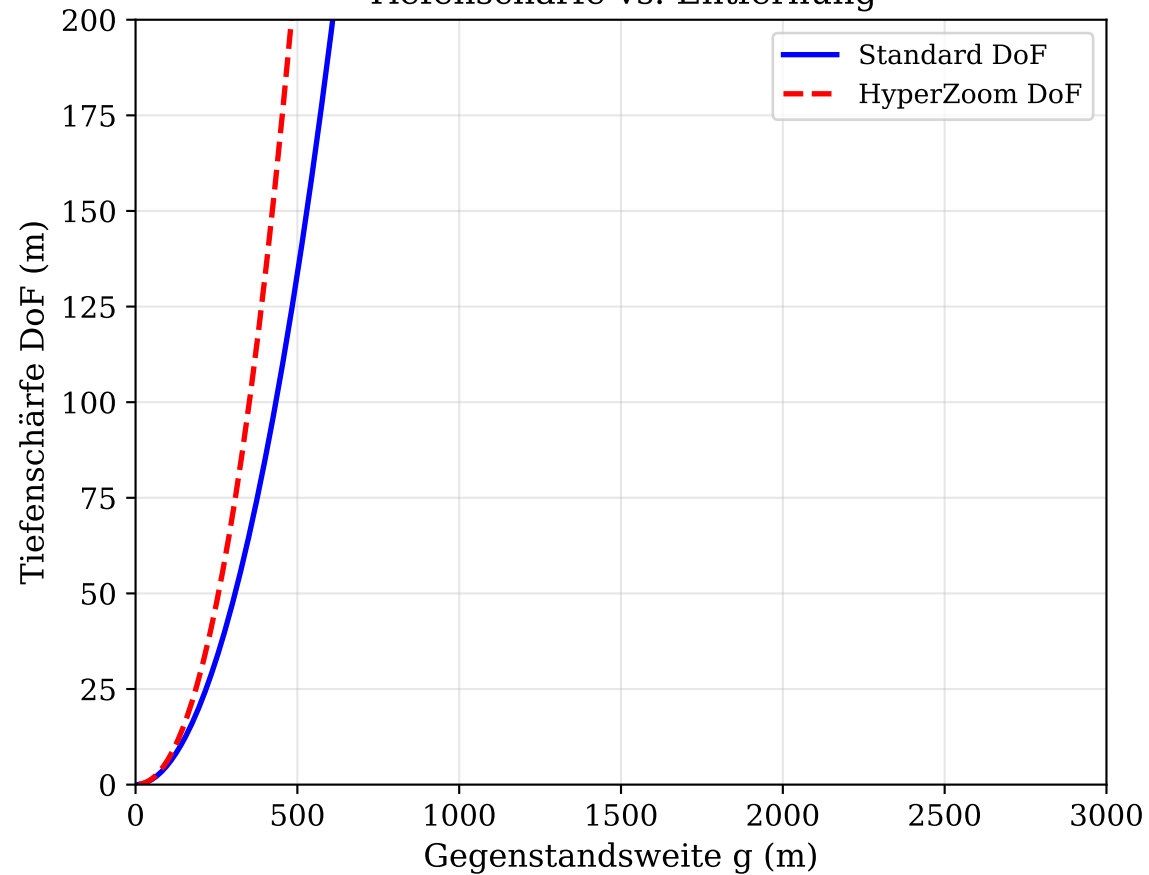
Tiefenschärfe vs. Entfernung
