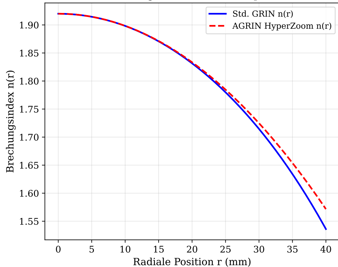
Brechungsindex-Gradientenprofil
