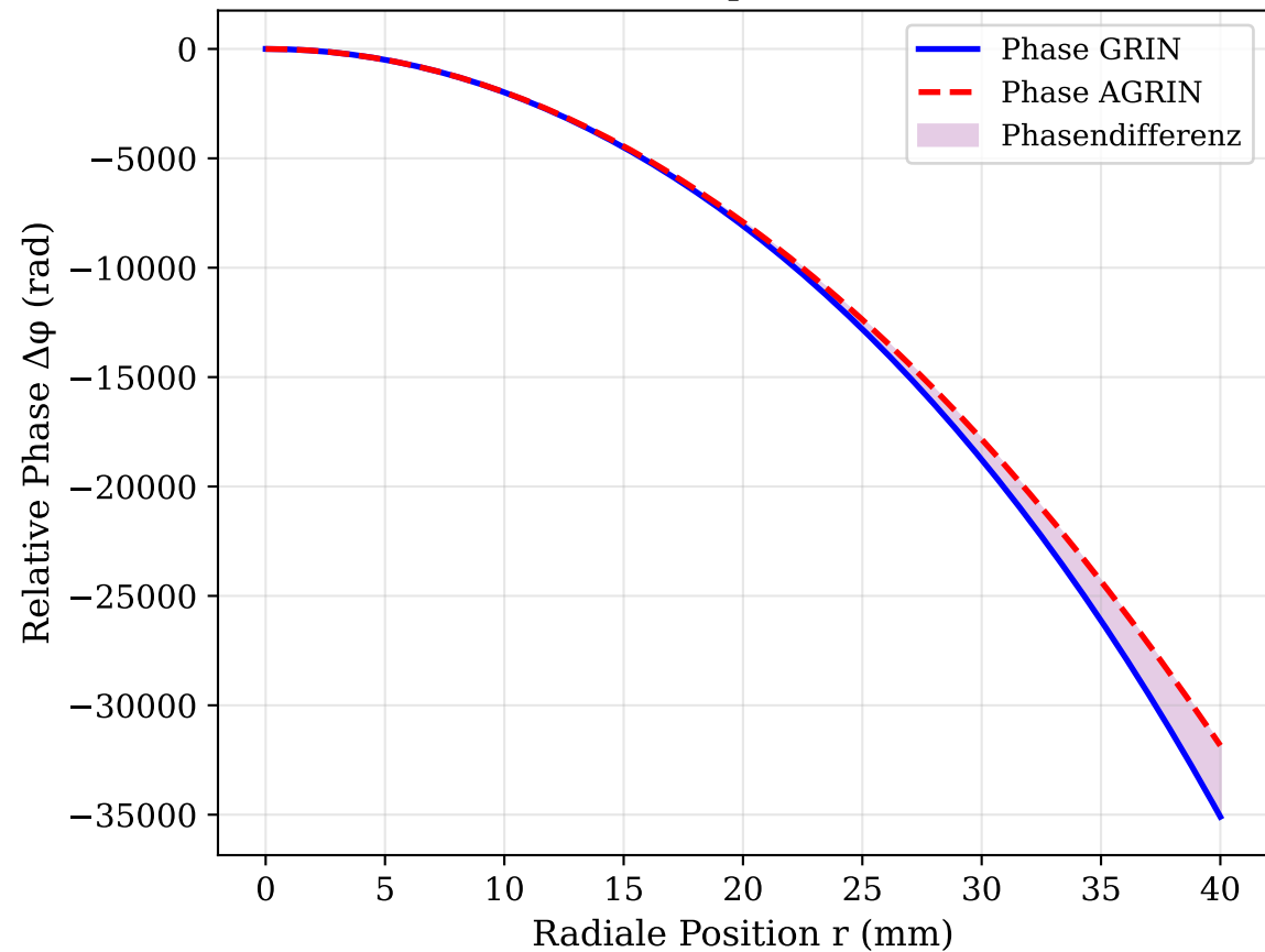
Wellenfrontphasen-Profil
