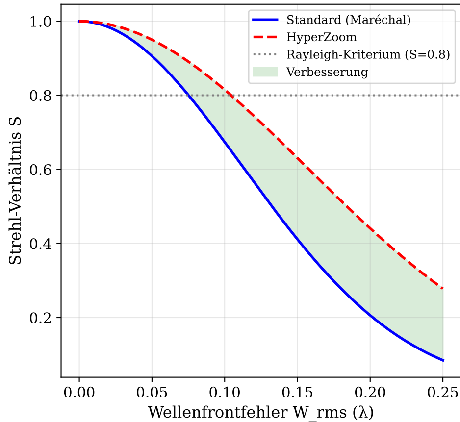
Strehl-Ratio vs. Wellenfrontfehler
