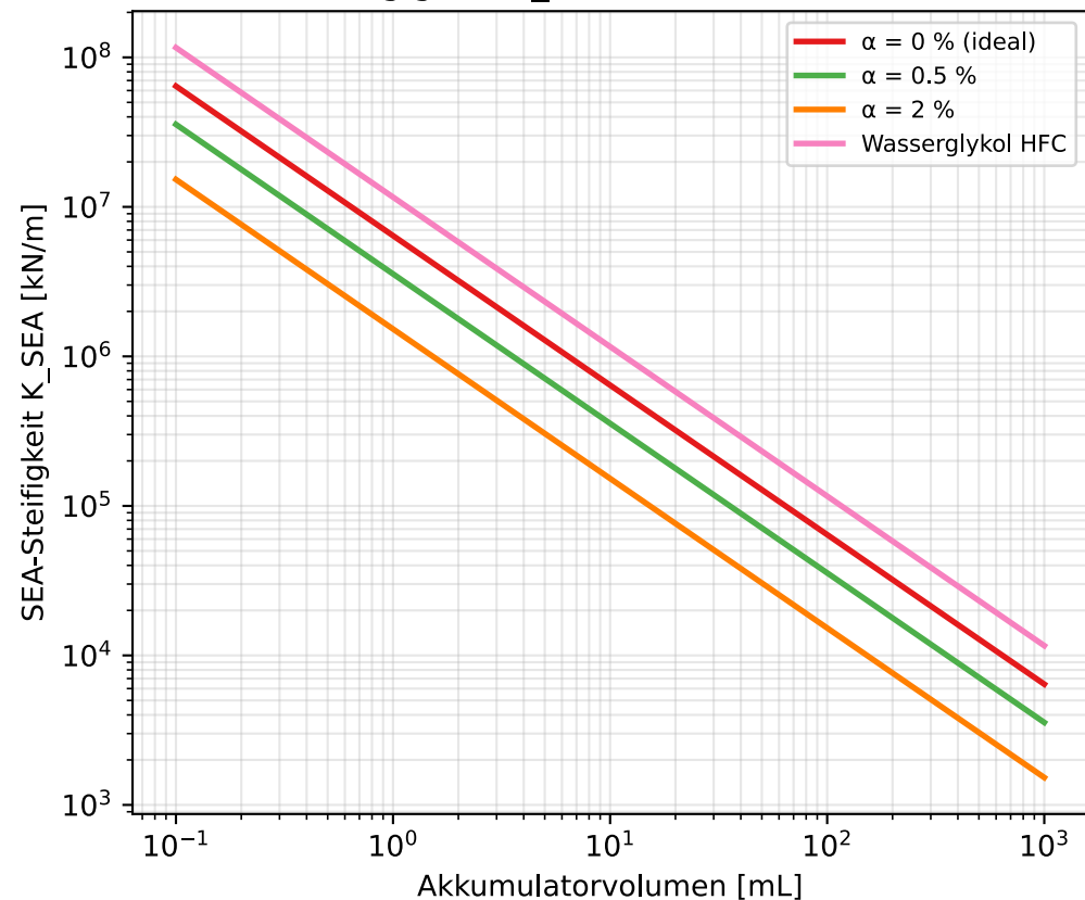
Abhängigkeit K_{SEA} vom Akkuvolumen
