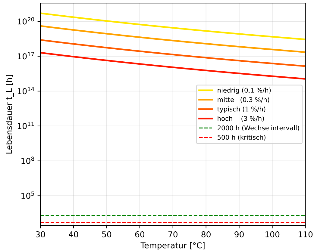
Arrhenius-Abfall der Öllebensdauer
