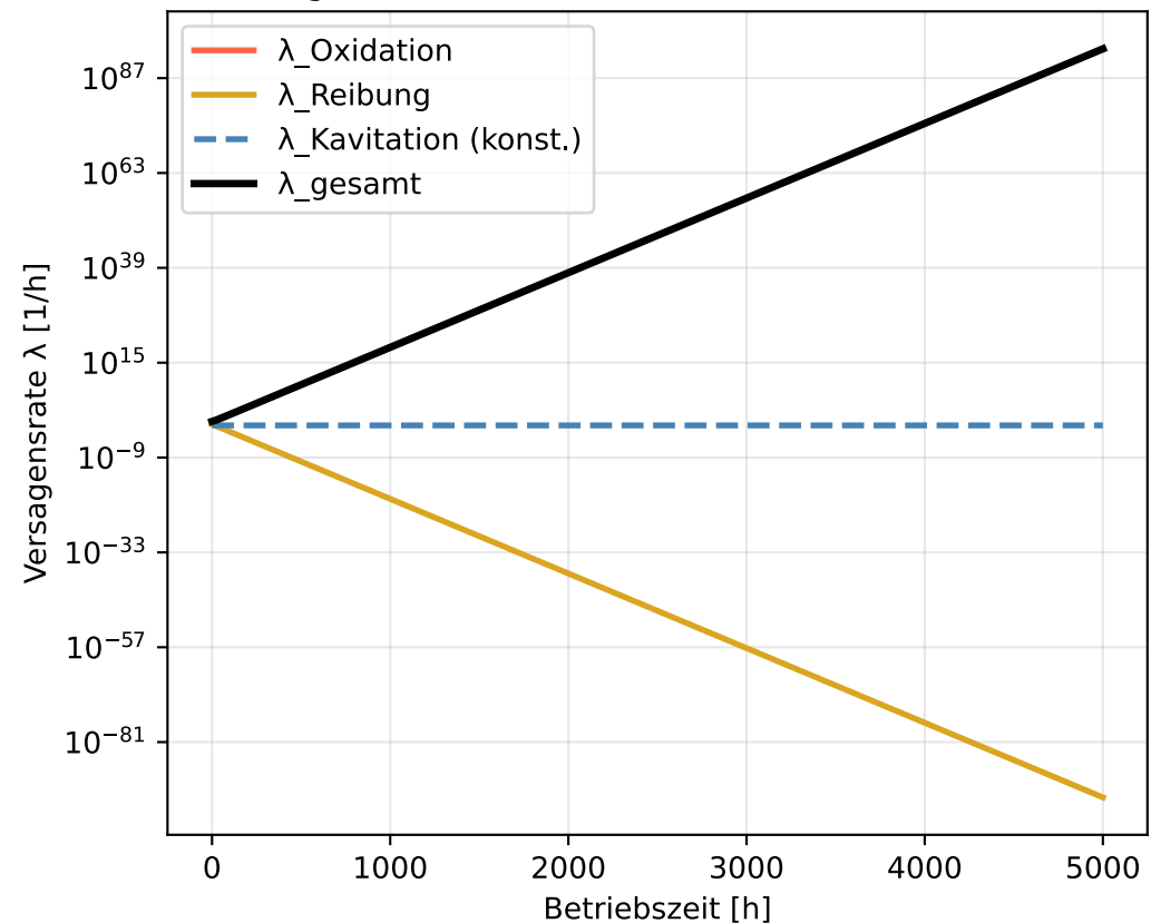
Versagensraten-Akkumulation (drei Mechanismen)
