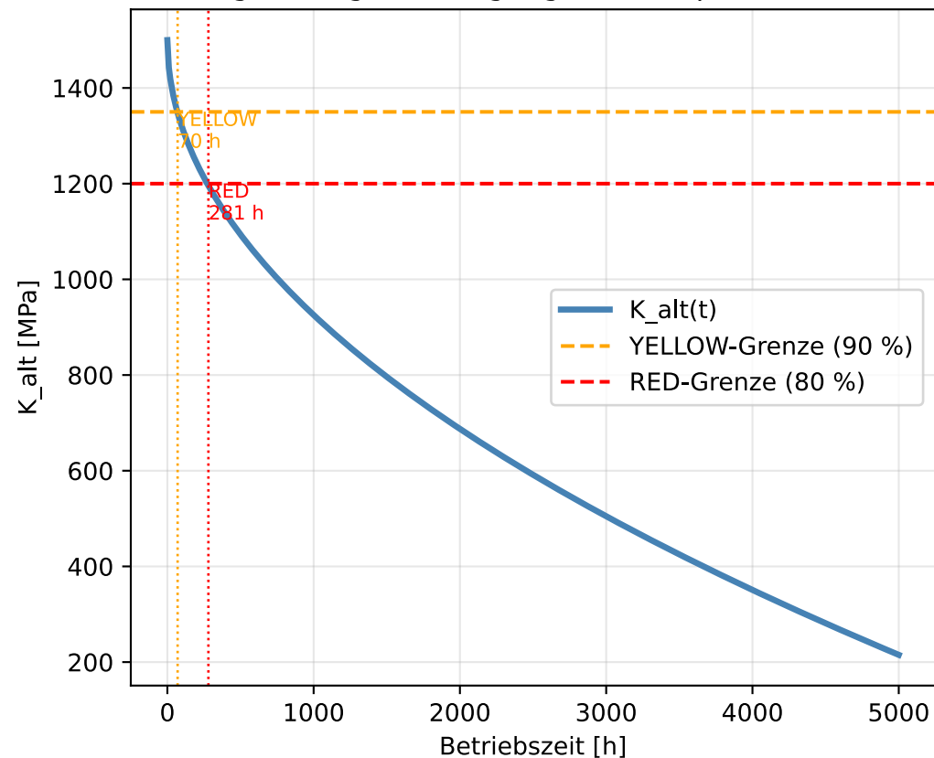
Alterungsbedingter Rückgang des Kompressionsmoduls
