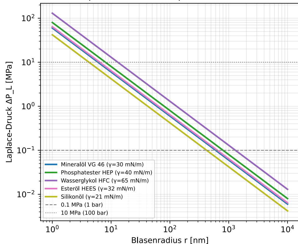
Laplace-Innendruck sphärischer Blasen
