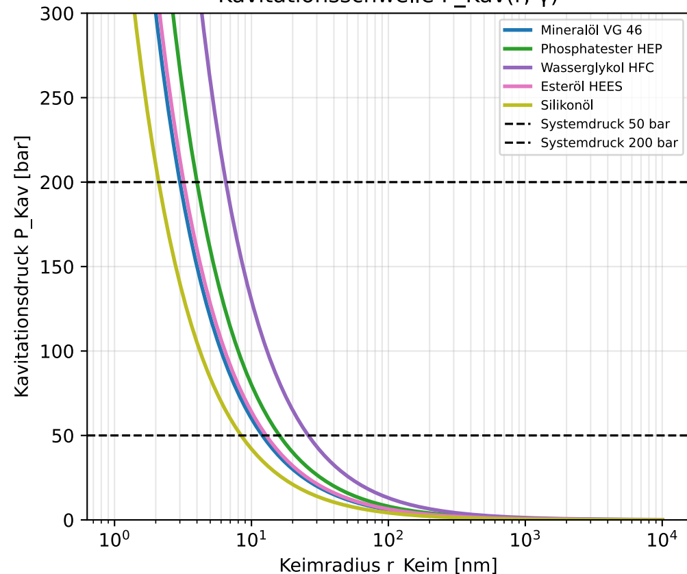
Kavitationsschwelle P_{Kav}(r, \gamma)
