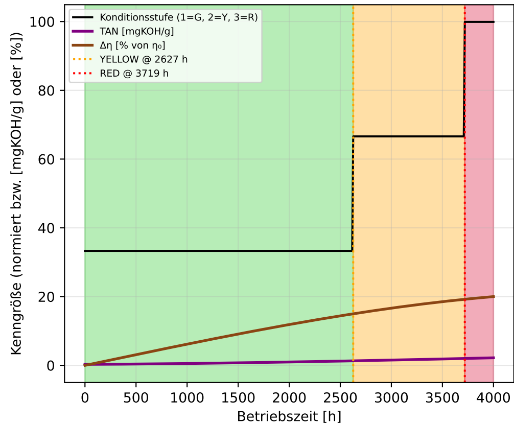
Konditionsindikator: TAN, \Delta\eta und Ampelbewertung
