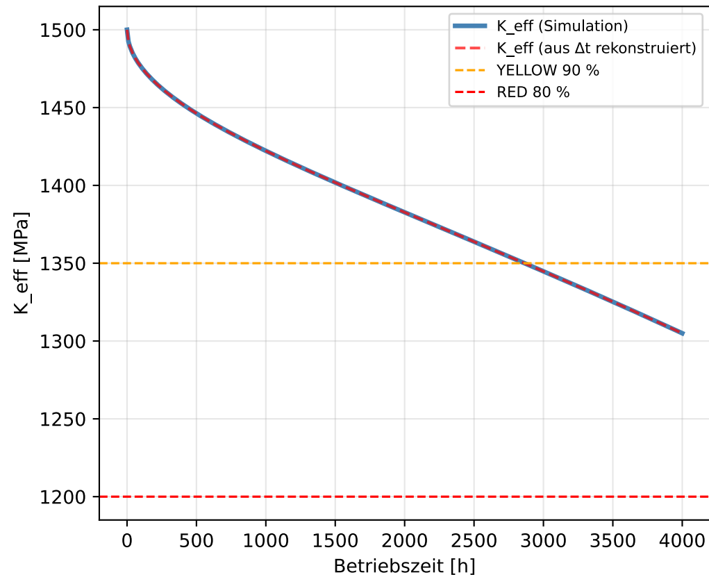
Kompressionsmodul über Betriebszeit
