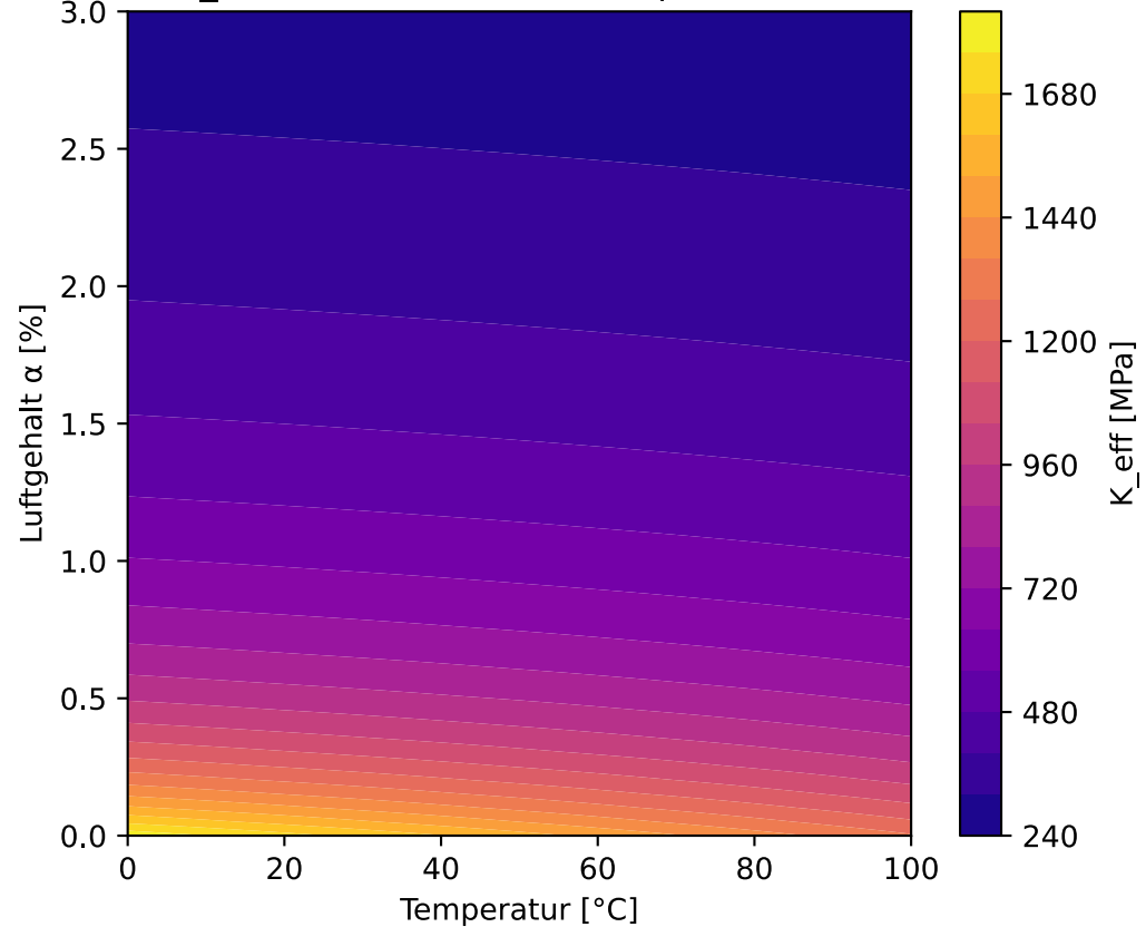
K_{eff}(T, \alpha) - Einflussraum ( p=100 bar)
