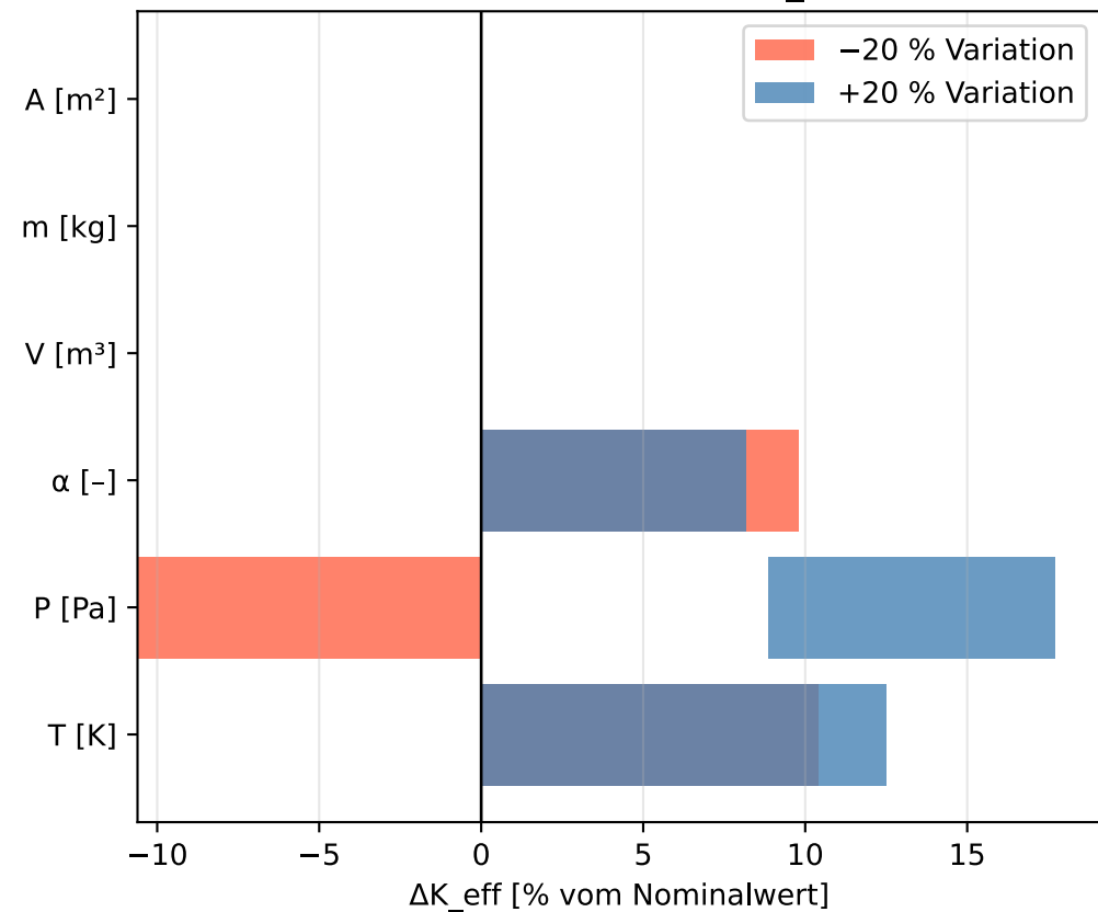
Tornado: Einfluss auf K_{eff}
