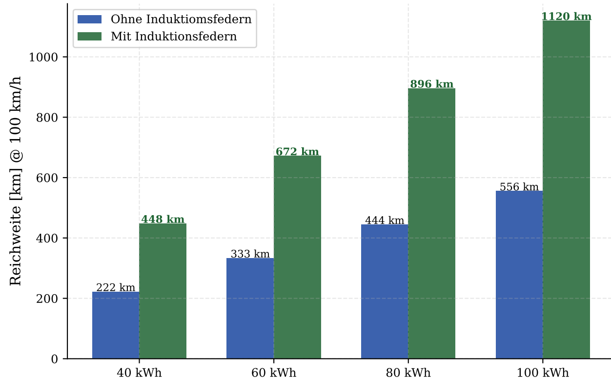
Reichweitengewinn E-Fahrzeug durch Induktionsfeder-Hilfsleistung
