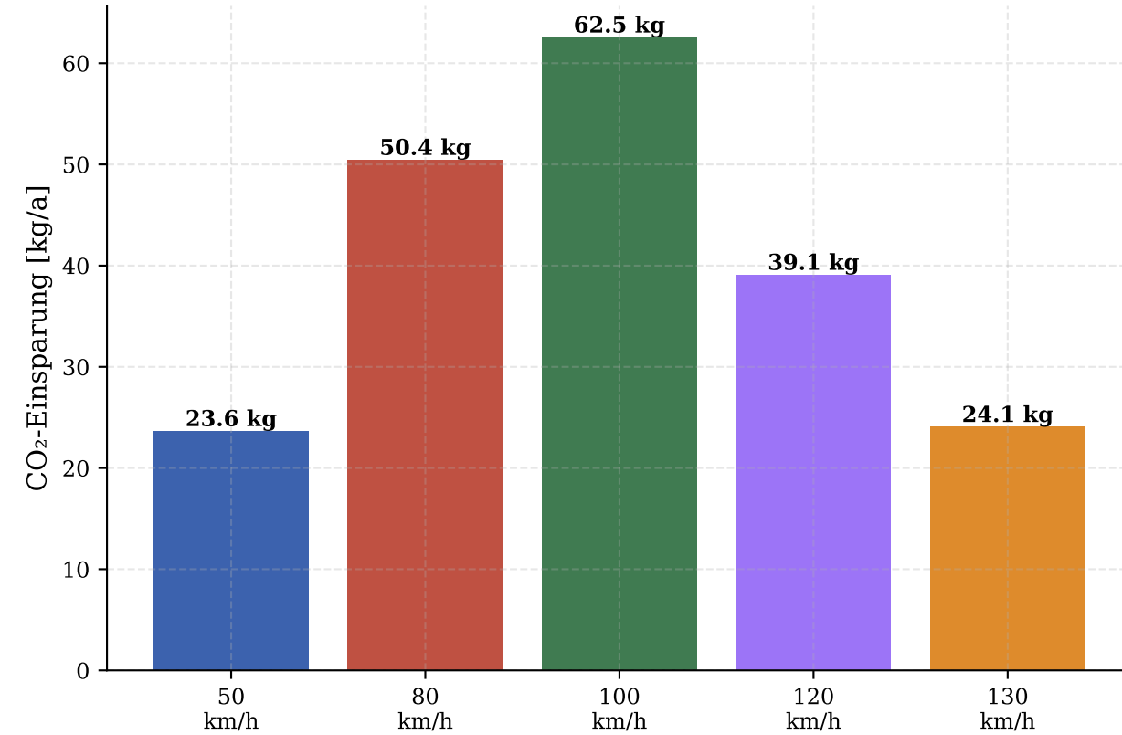
CO 2 -Einsparung durch Hilfsleistungs-Offset (15 000 km/a)
