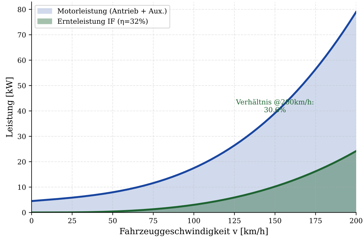
Reichweitengewinn E-Fahrzeug durch Induktionsfeder-Hilfsleistung
