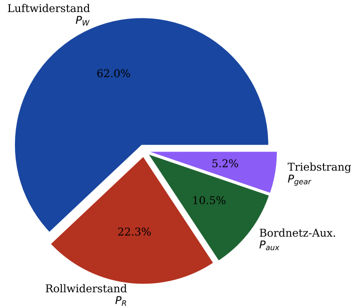
Leistungsverteilung bei 130 km/h (Gesamt: 28.6 kW)
