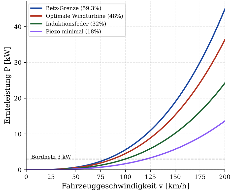
Ernteleistung bei voller Frontflächenausnutzung A = 0.72 m 2 (1.8 m \times 0.4 m)
