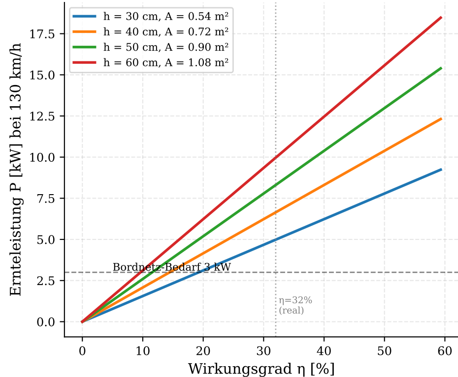
Ernteleistung vs. Wirkungsgrad bei verschiedenen Fronthöhen
