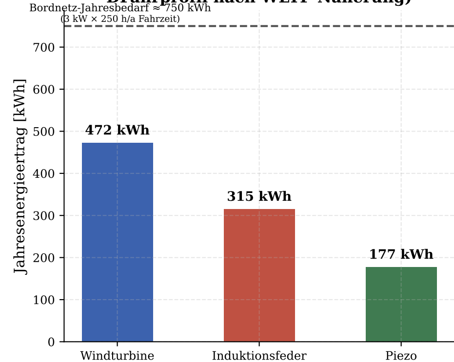
Jährlicher Energieertrag (15 000 km/a, D Fahrprofil nach WLTP-Näherung)
