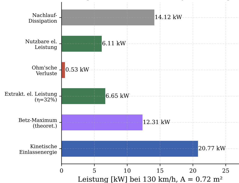
Energiefluss-Bilanz (Sankey-Näherung)
