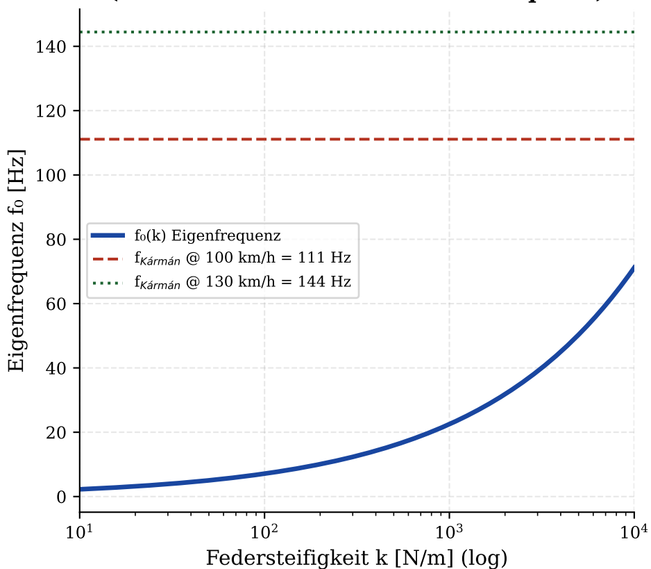
Optimale Federsteifigkeit (Resonanz mit Kármán-Wirbelfrequenz)
