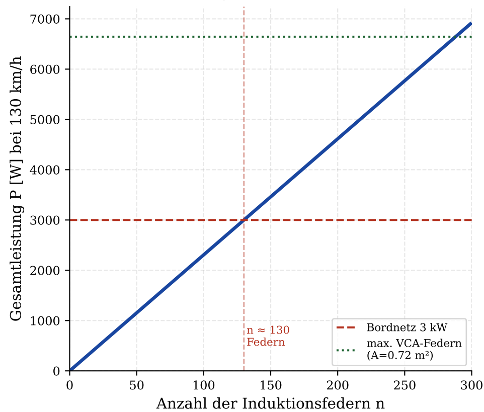
Array-Leistung vs. Federanzahl ( A_F = 5 \times 5 \text{ cm}^2 )
