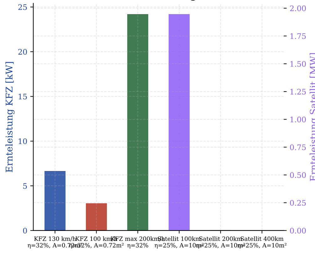
Vergleich aller Szenarien (Ernteleistung)
