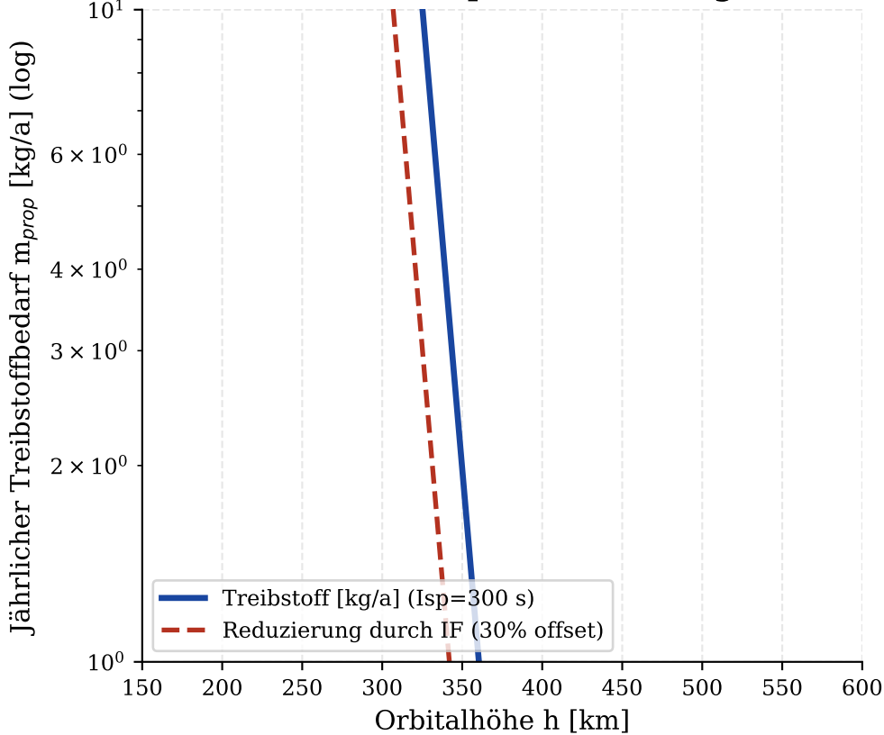
Jährlicher Treibstoffbedarf unter atmosph. Abbremsung
