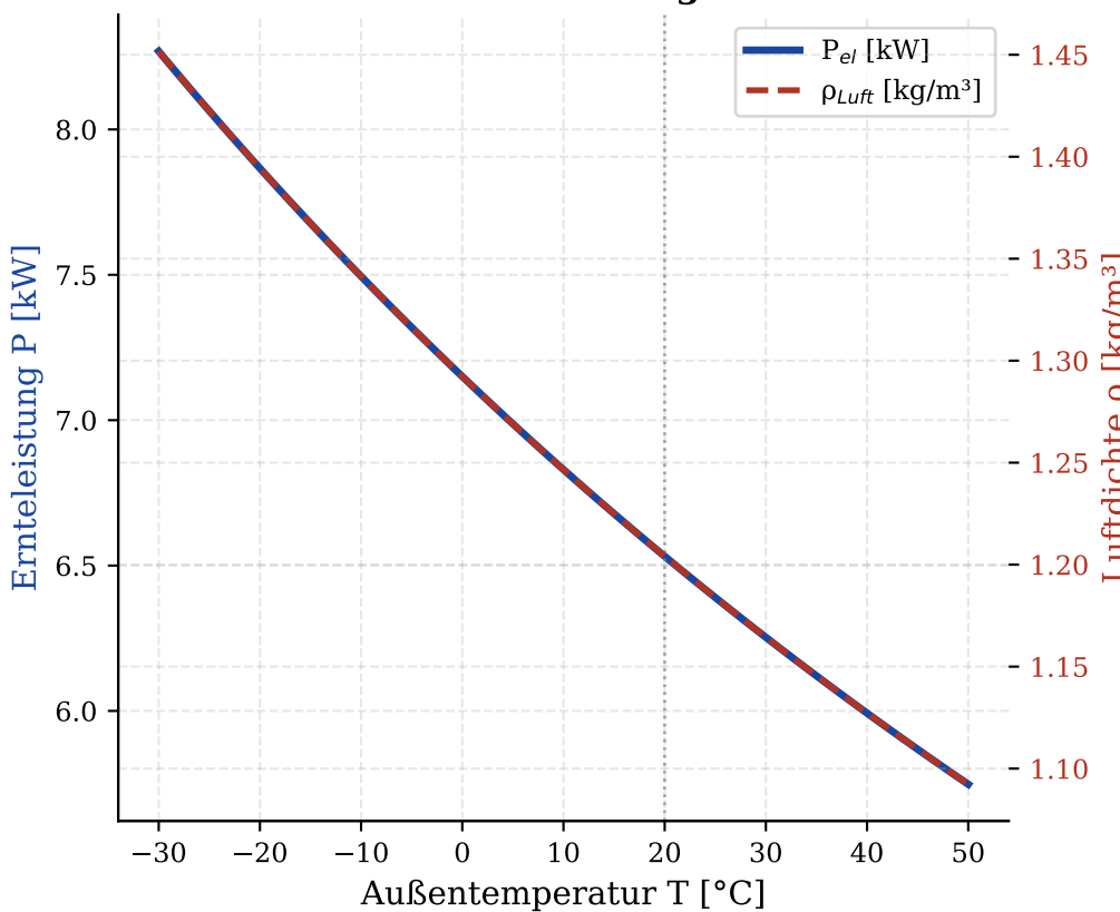
Temperaturabhängigkeit der Ernteleistung
