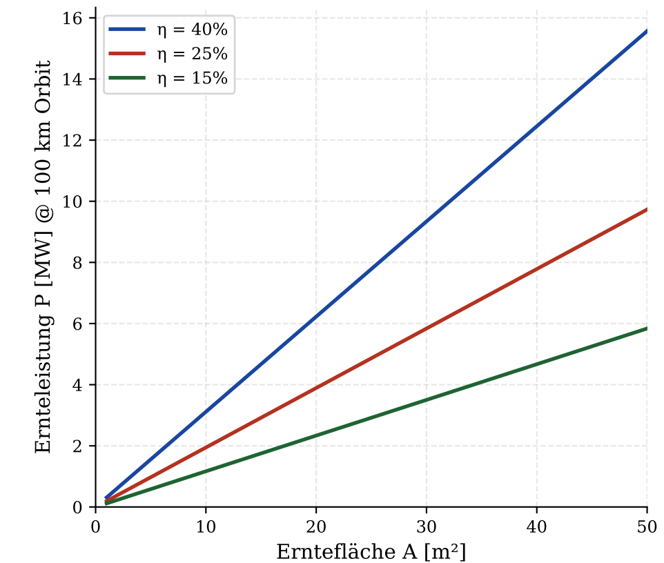
Satelliten: Ernteleistung als Funktion der Kollektorfläche
