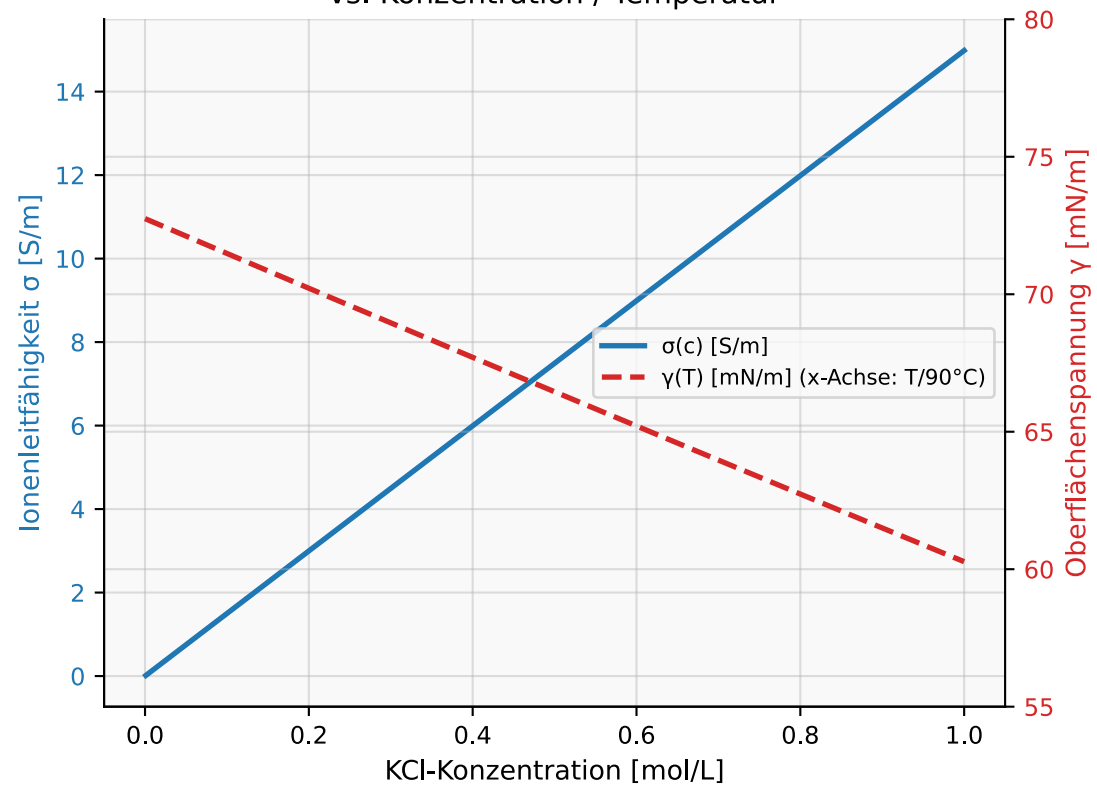
Ionenleitfähigkeit & Oberflächenspannung vs. Konzentration / Temperatur
