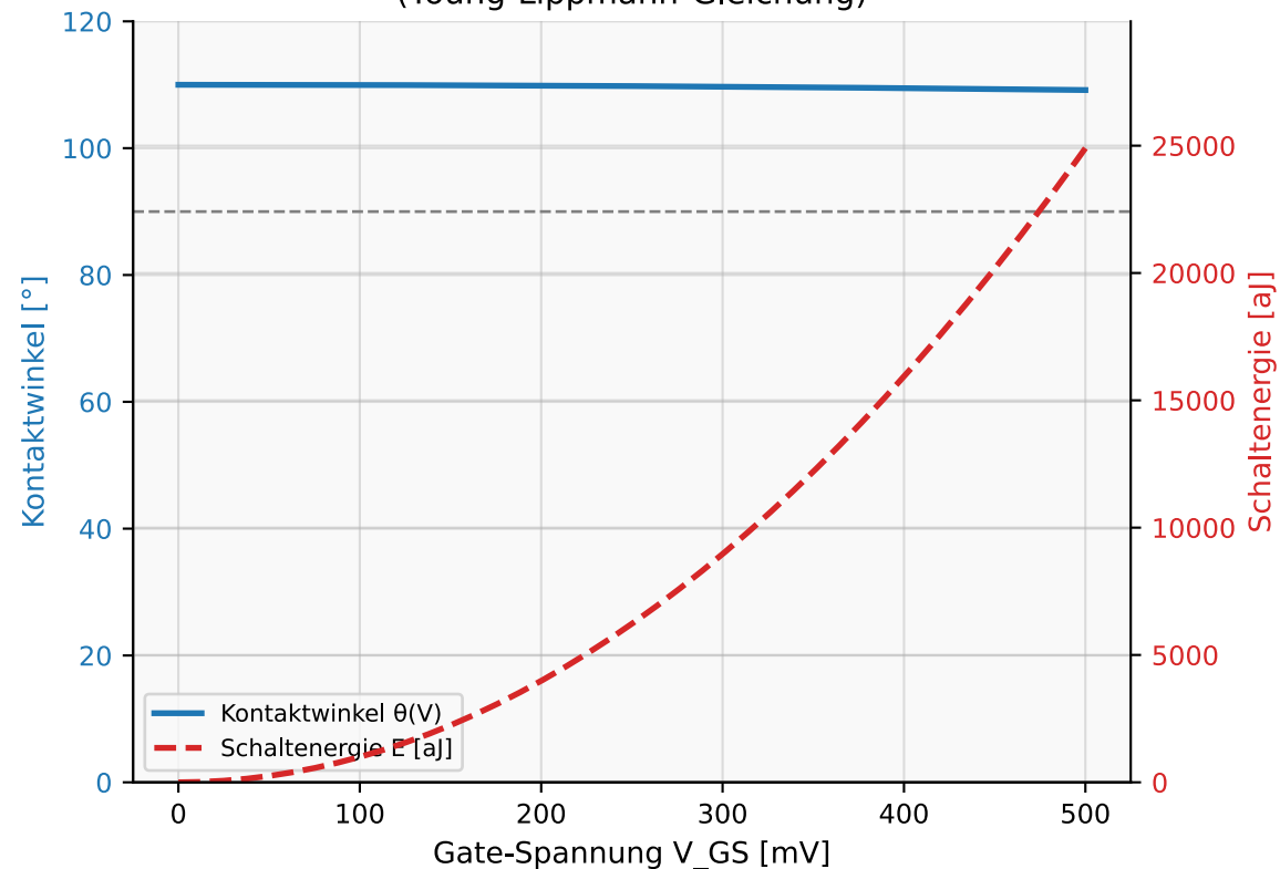
EWOD: Kontaktwinkel & Schaltenergie (Young-Lippmann-Gleichung)
