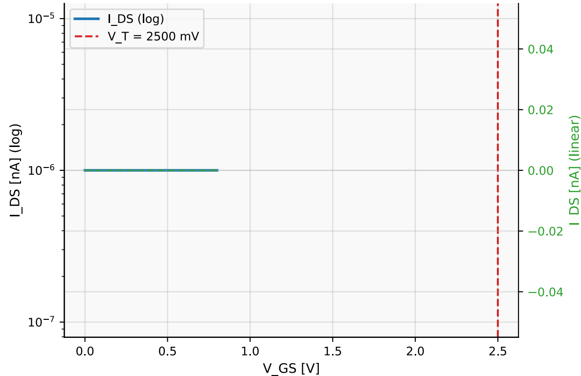
Übertragungskennlinie I_{DS}(V_{GS}) V_{DS} = 50 \text{ mV}
