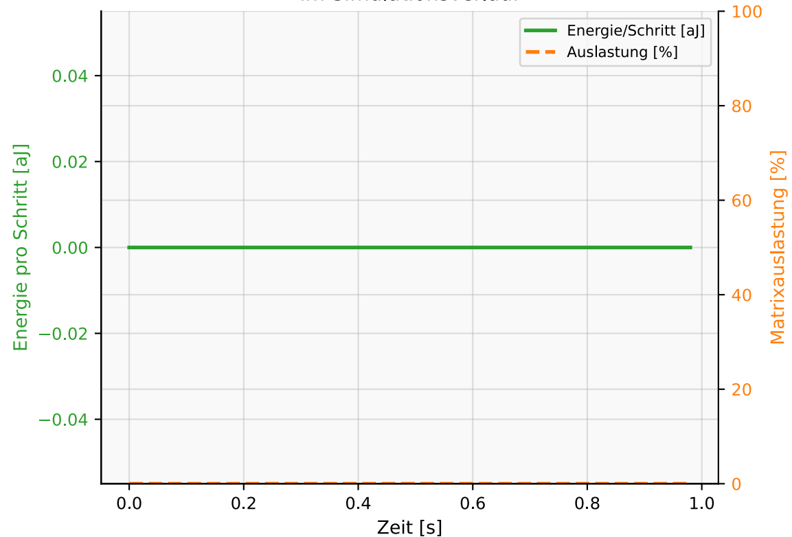
Energieverbrauch & Matrixauslastung im Simulationsverlauf
