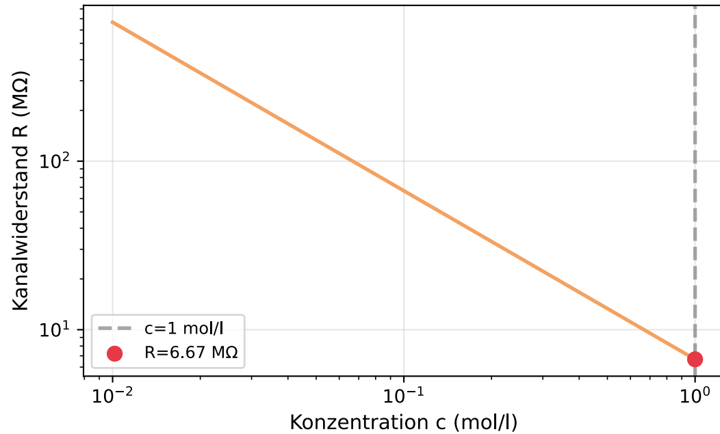
R(c) : Widerstand vs. KCl-Konzentration ( L=1\mu\text{m} , A=100\times 100\text{nm}^2 )
