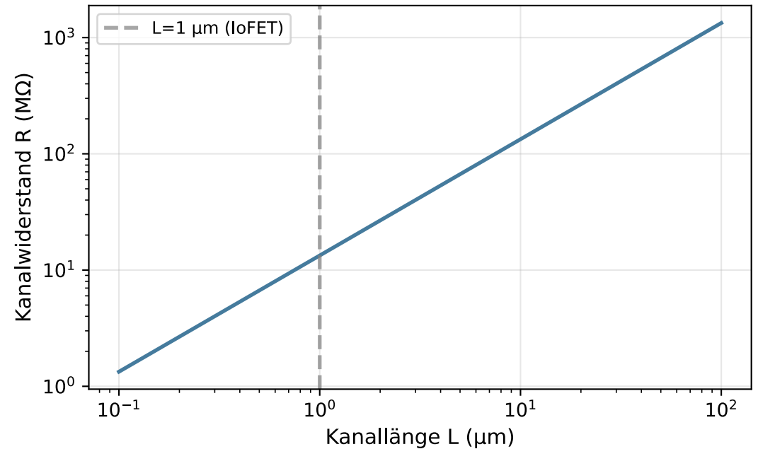
R(L) : Widerstand vs. Kanallänge ( c=0.5\text{ mol/l} , A=100\times 100\text{nm}^2 )
