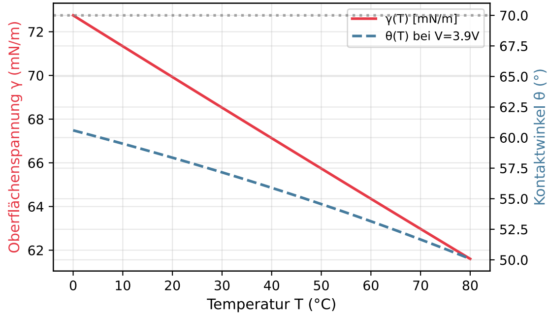
\gamma(T) und \theta -Drift ohne Kompensation (Drift: 10.5^\circ )
