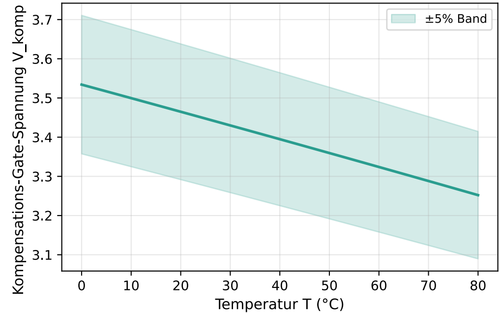
V_{\text{komp}}(T) für konstantes \theta=70^\circ
