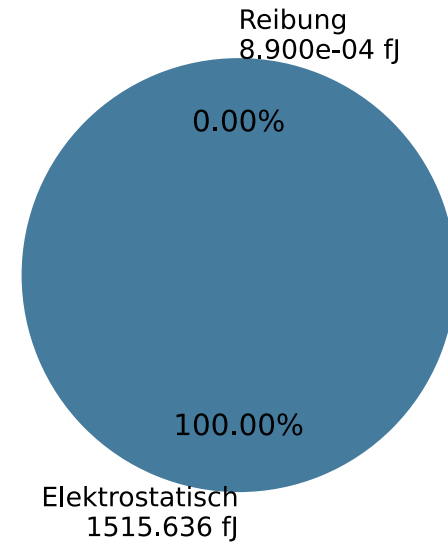
Energieanteile bei v = 1 \mu\text{m/ms} CMOS-Ratio: 0.1x
