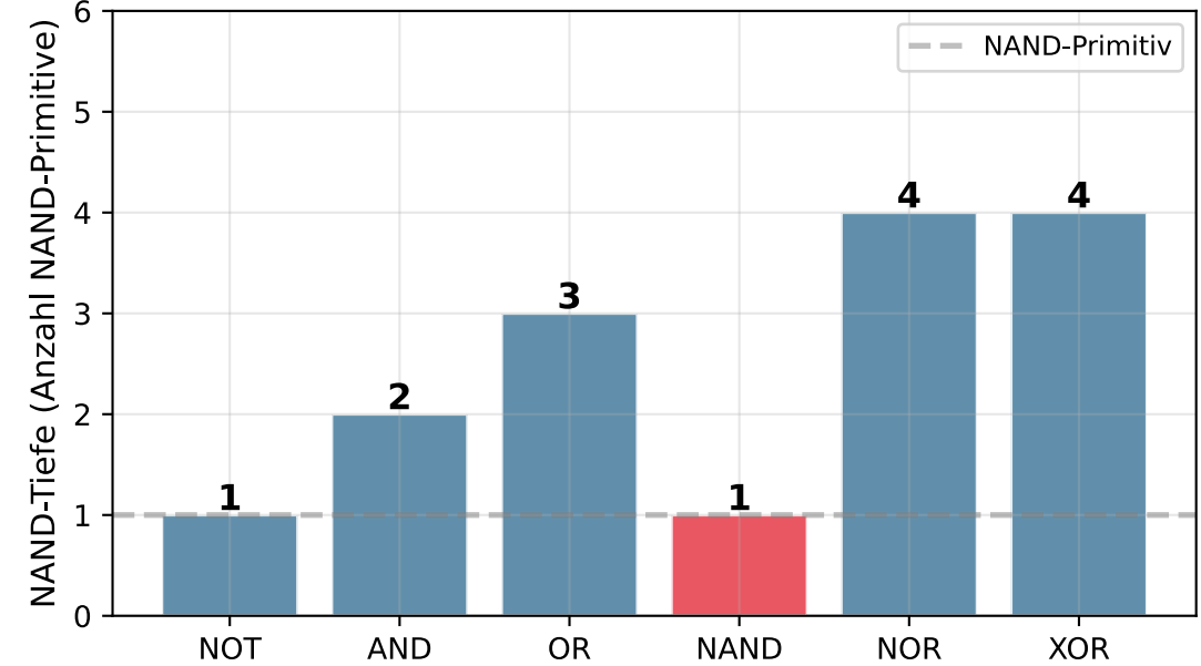
NAND-Zerlegungstiefe aller Logikgatter (NAND ist Primitiv der Tiefe 1)
