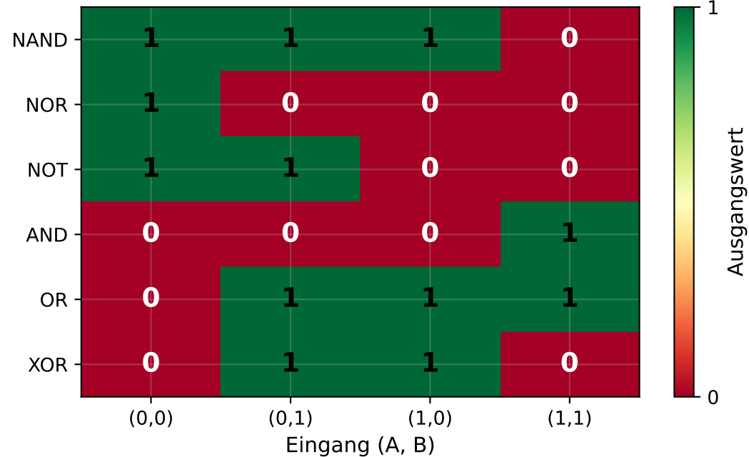
Wahrheitstafeln aller Logikgatter (Grün=1, Rot=0)
