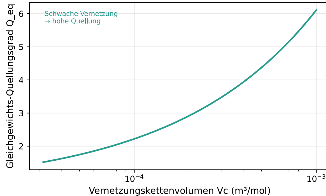
Flory-Rehner: Q_{eq}(V_c) - Vernetzungsdichte ( \chi=0.25 , Ethanol)
