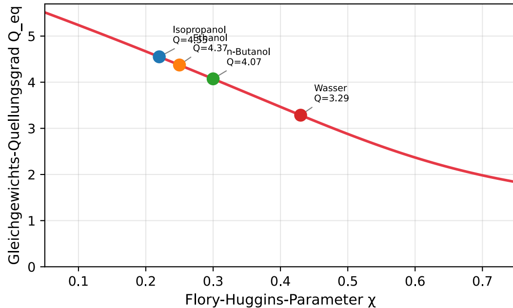
Flory-Rehner: Q_{eq}(\chi) - Lösungsmiteleinfluss ( V_m=1.8e-5 \text{ m}^3/\text{mol} , V_c=5e-4 \text{ m}^3/\text{mol} )
