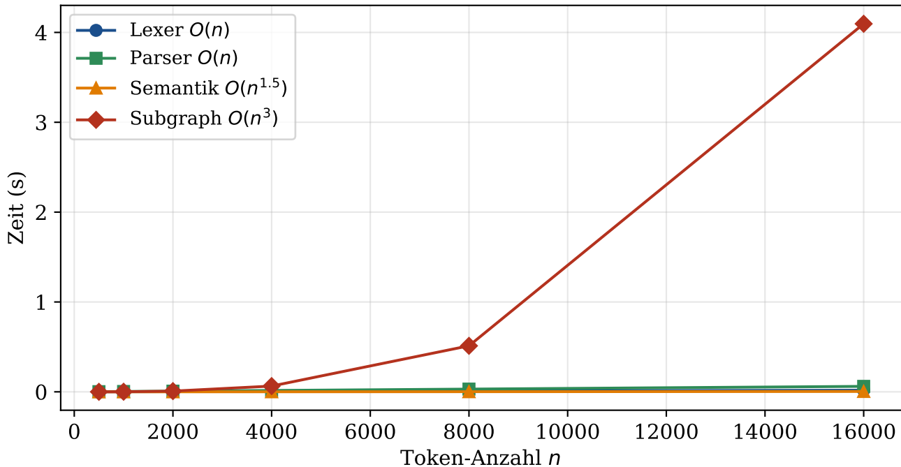
Laufzeitvergleich der Compilerphasen
