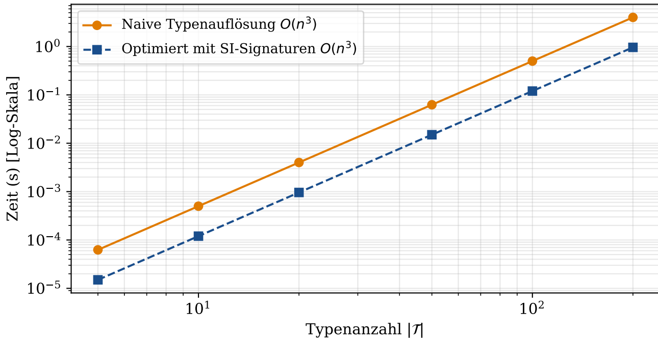
Reduktionszeit: Typabhängigkeitsgraph (TAP)
