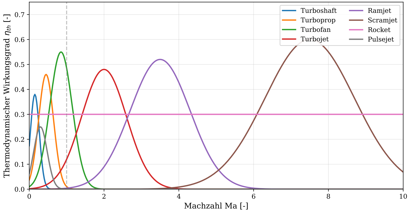
Thermodynamischer Wirkungsgrad verschiedener Strahltriebwerkstypen
