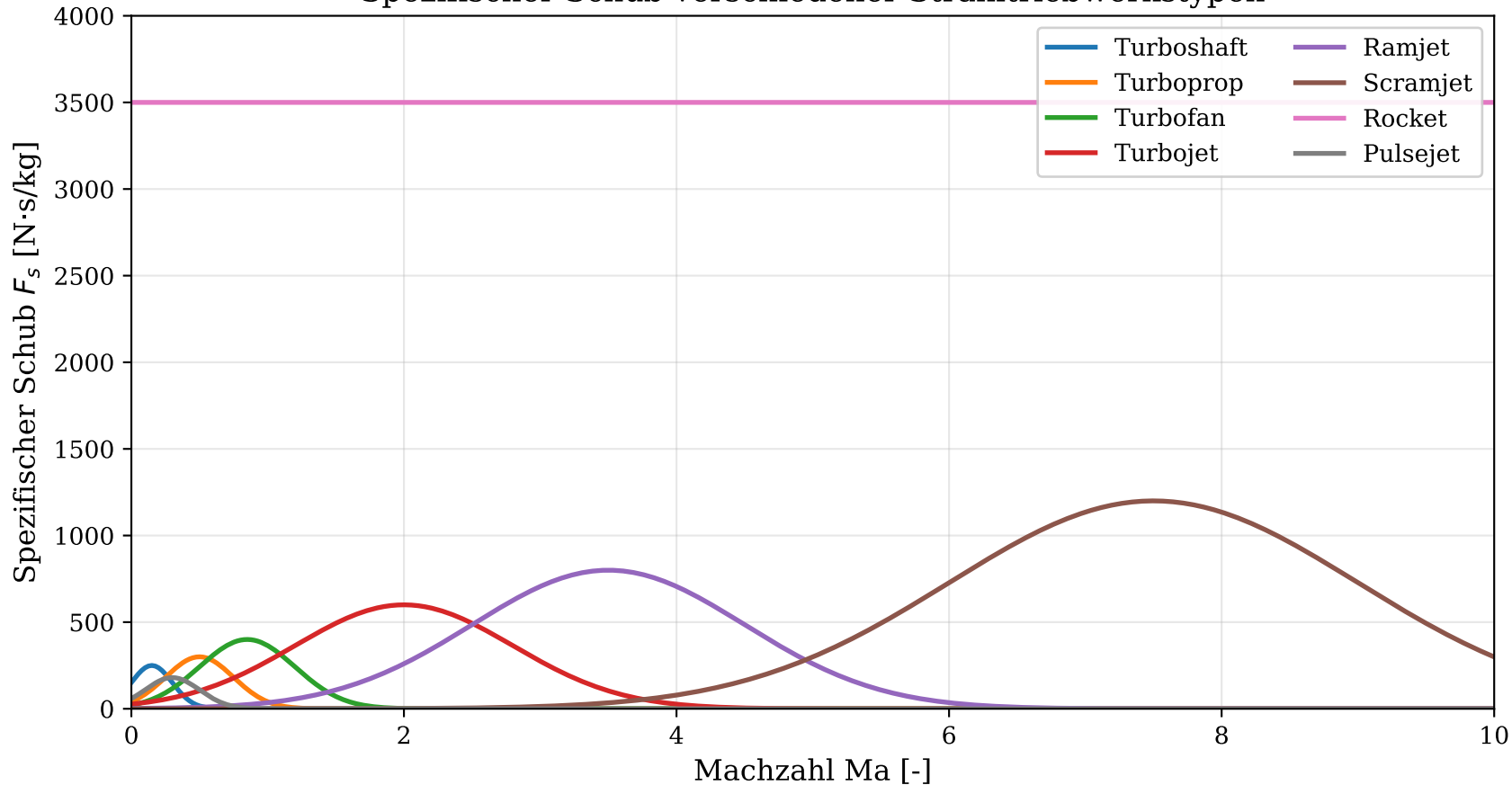
Spezifischer Schub verschiedener Strahltriebwerkstypen
